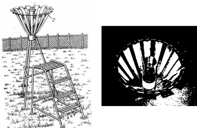
Рис. 18. Осадкомер Третьякова О-1
