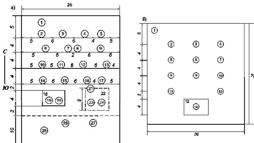
Рис. 1. План размещения оборудования и приборов на метеорологической площадке (расстояния указаны в метрах)
