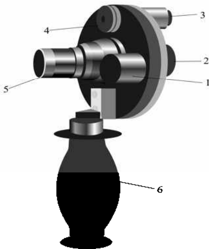
Рис. 25. Поляризационный измеритель видимости М-53А
