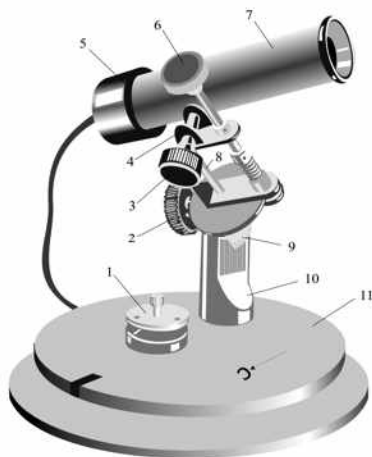
Рис. 3. Актинометр термоэлектрический АТ-50:
