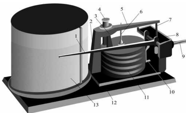
Рис. 35а. Барограф метеорологический М-22АН
