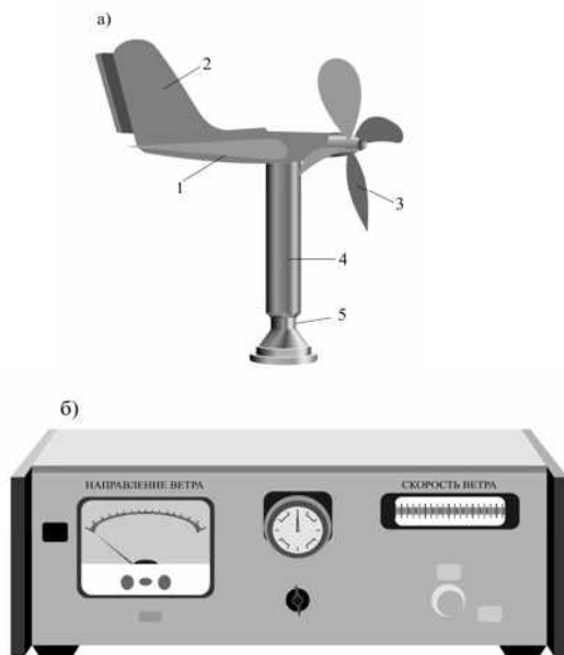
Рис. 38. Анеморумбометр М-63М-1
