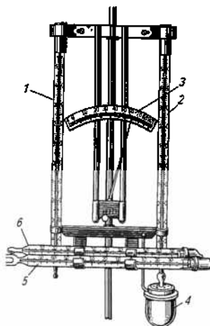
Рис. 7. Гигрометр М-19
