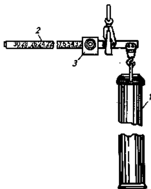
Рис. 23а. Снегомер весовой 1 — металлический градуированный цилиндр, 2 — металлическая линейка со шкалой, 3 — гири безмена
