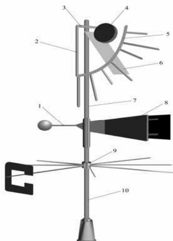
Рис. 39. Флюгер Вильда
