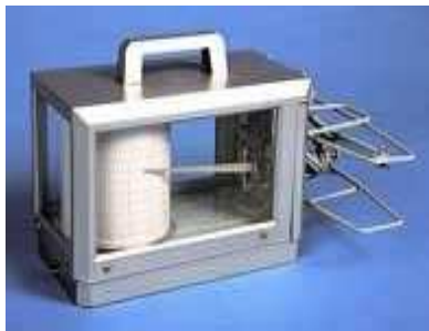
Рис. 8. Гигрограф М-21АС (общий вид)
