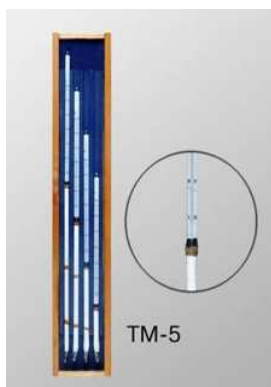
Рис. 12. Термометр метеорологический стеклянный типа ТМ-5
