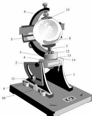
Рис. 2. Гелиограф универсальный модели ГУ-1
