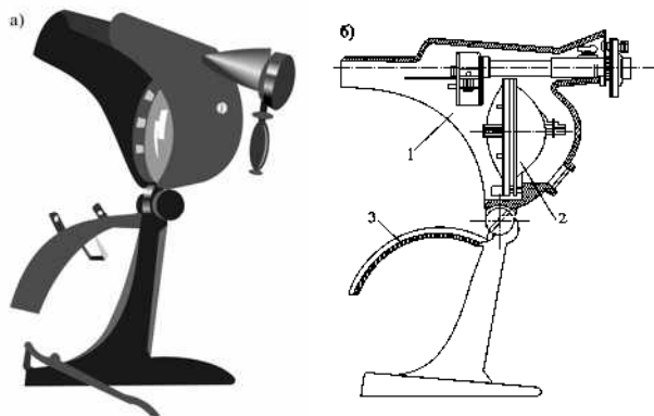
Рис. 26. Нефелометрическая установка обратного рассеяния М-71
