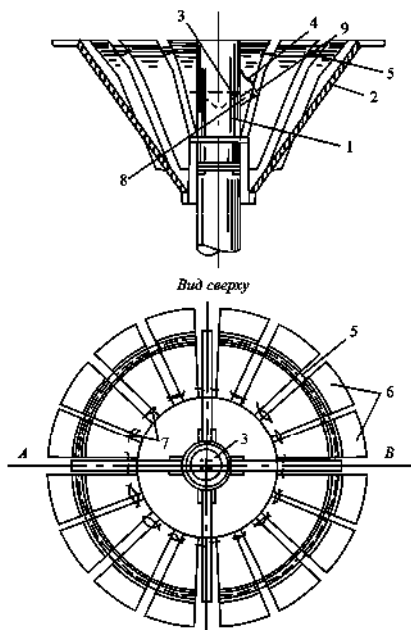
Рис. 18 а. Осадкомер О-1:
