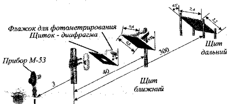
Рис. 30. Схема размещения оборудования при наблюдениях по комплексному способу
