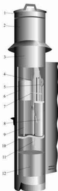
Рис. 20. Плувиограф П-2
