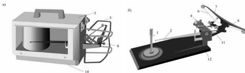
Рис. 8а. Гигрограф М-21АС
