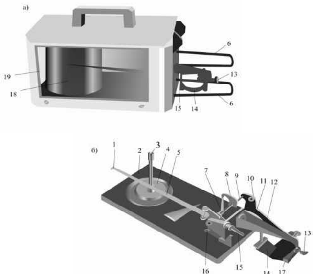
Рис. 6а. Термограф метеорологический М-16АС
