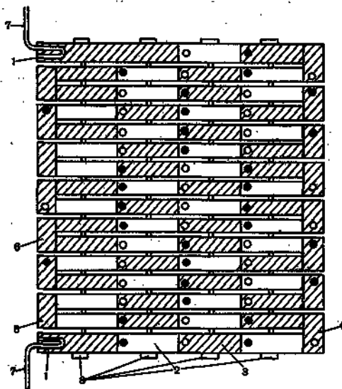
Рис. 6. Термобатарея пирометра: 1, 7 — полюса термобатарей, 2 — константановые полоски, 3 — манганиновые полоски, 4, 5, 6 — перемычки, 8 — охлаждающие ребра
