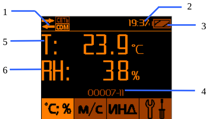
Рис.4 – Измерение температуры и влажности воздуха
