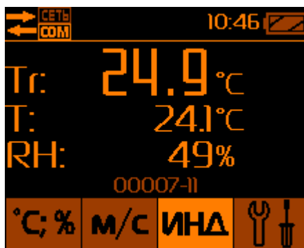
Рис.17 – Режим определения результирующей температуры
