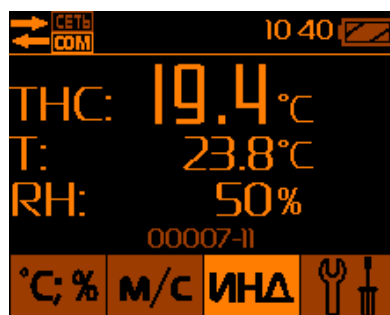
Рис.13 – Определение ТНС-индекса с подключённым датчиком «чёрный шар»
