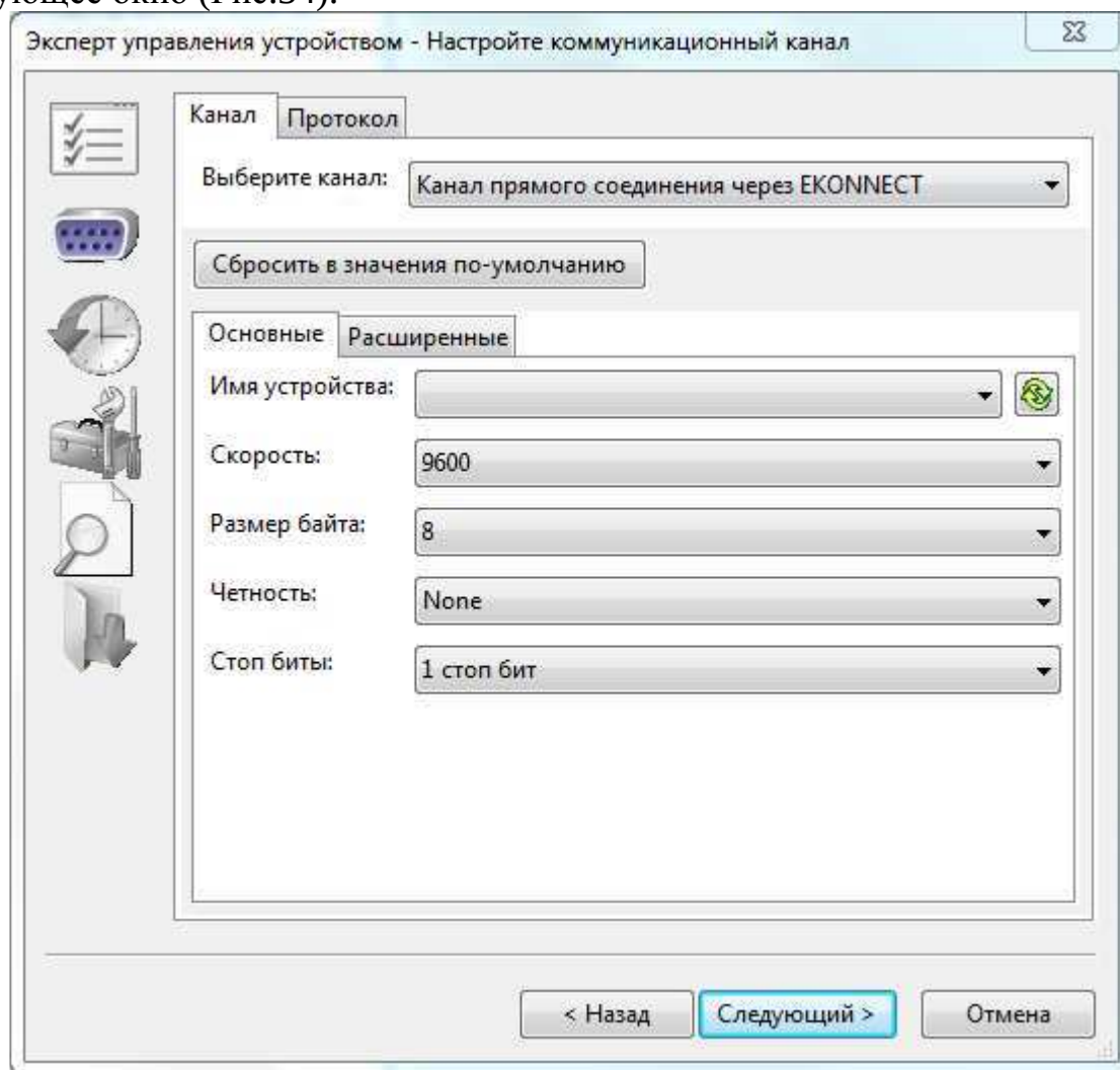
Рис.34 – Настройка коммуникационного канала с БОИ-01
