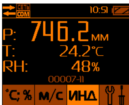
Рис.21 – Режим измерения атмосферного давления
