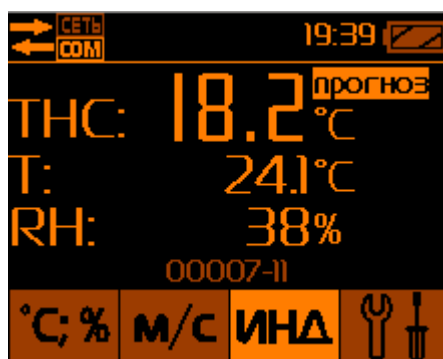
Рис.14 – Прогнозный расчёт ТНС-индекса при отсутствии подключённого «чёрного шара»
