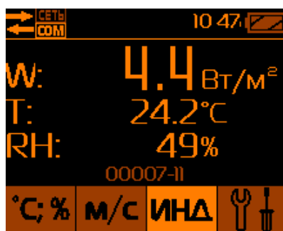
Рис.18 – Режим определения интенсивности теплового облучения
