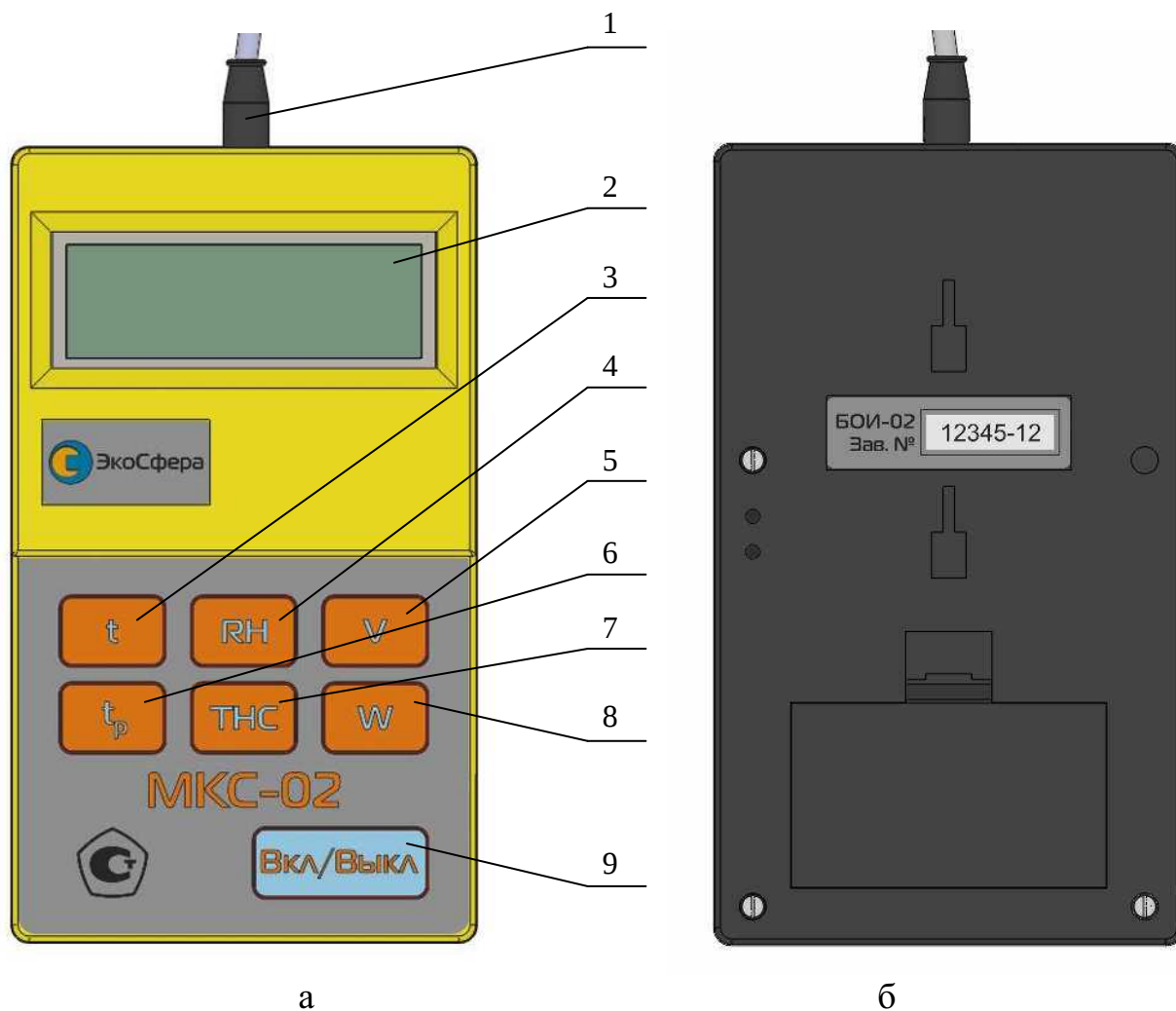
Рис. 1 – Внешний вид блока отображения информации MKC-02 (а - лицевая сторона, б – тыльная сторона)
