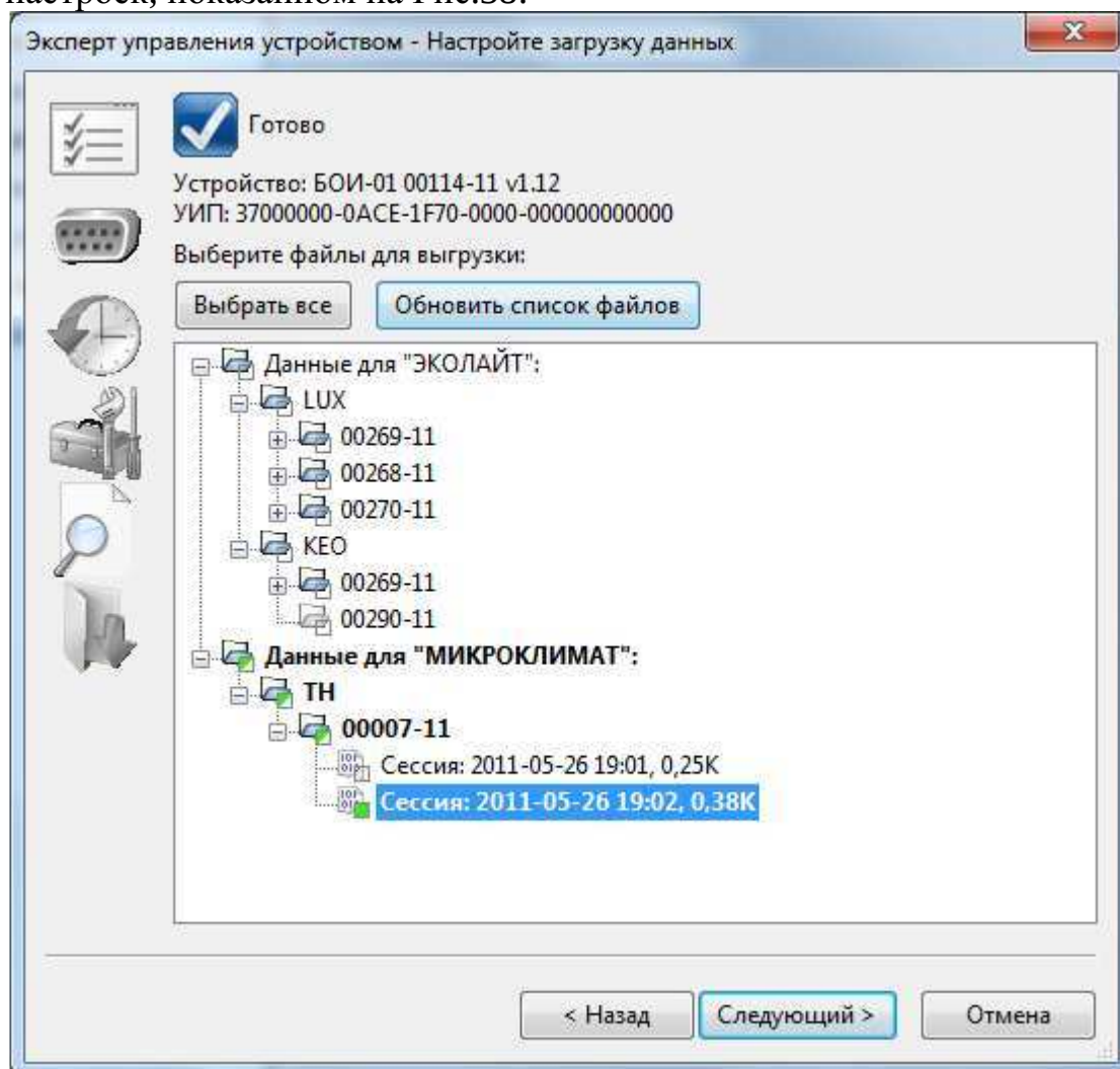
Рис.38 – Окно настройки загрузки данных из БОИ-01
