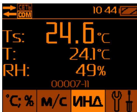
Рис.16 – Режим отображения температуры «чёрного шара»
