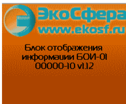
Рис.2 – Стартовая заставка
