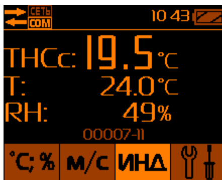
Рис.15 – Определение ТНС-индекса с солнечной нагрузкой
