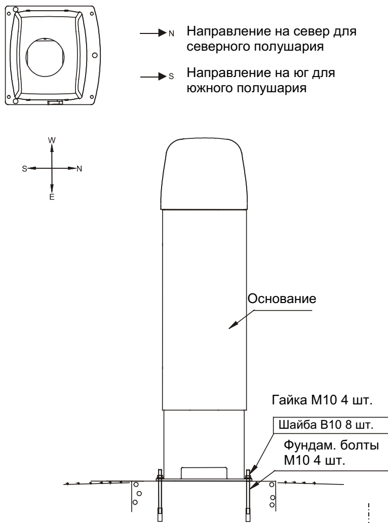
Рисунок 6 Установка экрана
