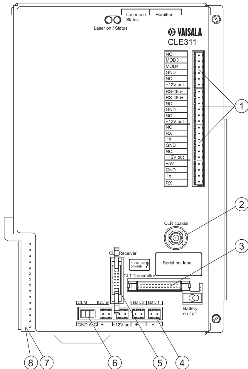
Рисунок 11 Внутренние соединения
