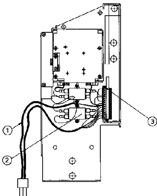
Рисунок 22 Оптическая рама с кабельным жгутом
