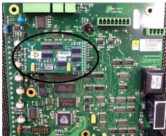
Рисунок 24 DMX501.
