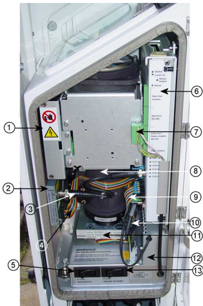
Рисунок 17 Облакомер CL31
