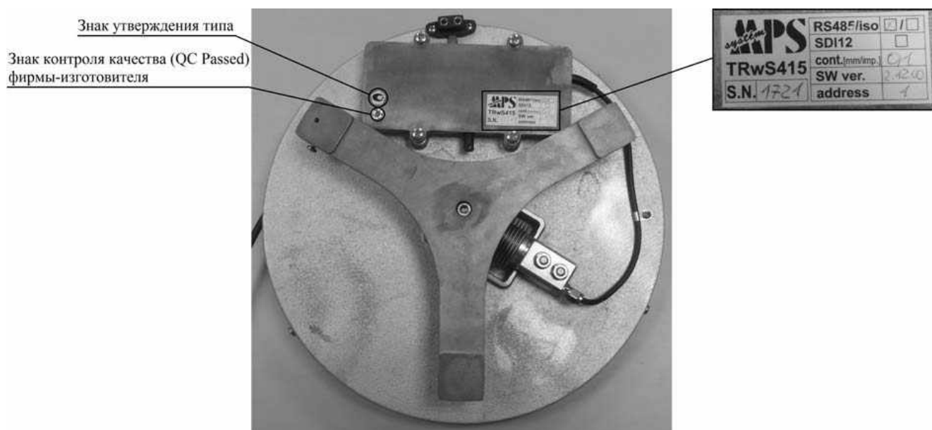
Рисунок 2 - Внешний вид станины и крышки корпуса электронного оборудования
