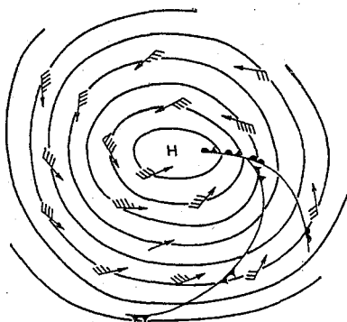
Рис. 24. Фронтальный циклон в стадии окклюдированного циклона.
