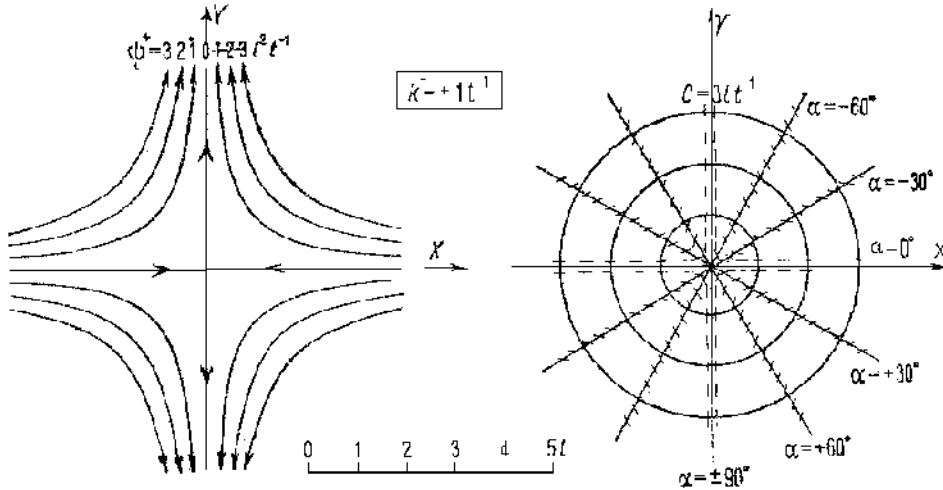
Рис. 3.1. Линии тока в линейном деформационном поле u = -ax, v = ay (слева); изотахи (окружности) и линии равных направлений (прямые, проходящие через центр) (справа).
