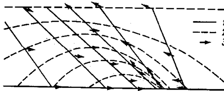
Рис. 3.7. Вертикальный разрез через зону фронта в горизонтальном деформационном поле при нулевом потенциальном вихре и жесткой верхней границе (Hoskins, Bretherton, 1972): 1 – изолинии X ; 2 – изолинии v ; 3 – векторы скорости в плоскости x, z .
