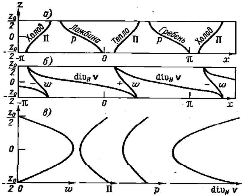
Рис. 2.8. Изменения фазы бароклинно-неустойчивых возмущений давления ( p ), энтропии ( \Pi ), вертикальных движений ( w ) и дивергенции ( div_H v ) в плоскости x, z (а, б) и распределение их амплитуд (абсолютных величин амплитудных функций) по высоте (в) в горизонтальном слое толщиной z_0 , по (Eady, 1949).
