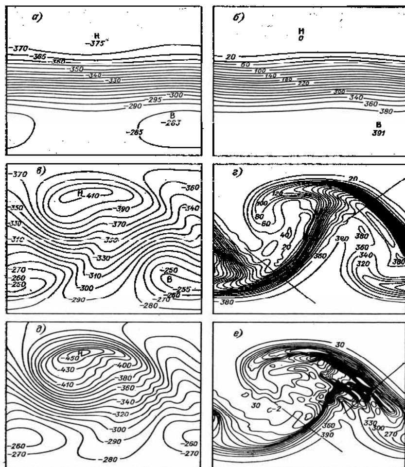
Рис. 2.16. Поле давления на нижнем уровне (а, в, д) и плавучести \theta' / \theta (б, з, е) в бароклинно- и баротропно-неустойчивой волне со временем удвоения 27 ч: а, б – начальное поле ( t = 0 ), разность давлений B - H = 21 гПа; в, з – квазигеострофическое решение, t = 144 ч, B - H = 21 гПа; д, е – решение полных уравнений, t = 144 ч, B - H = 45 гПа.
