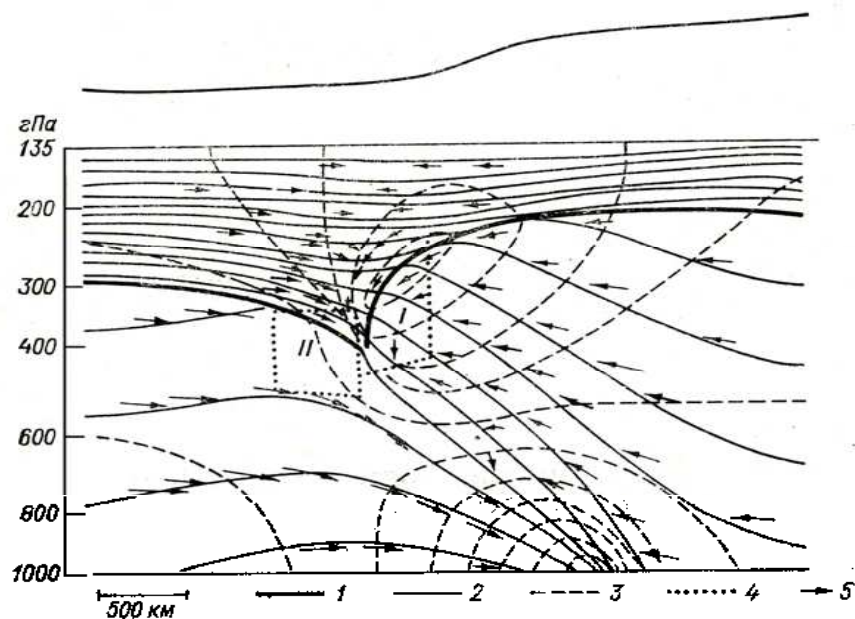
Рис. 3.8. Вертикальный разрез фронтальной зоны, полученный в двухслойной модели (Hoskins, 1971): 1 – тропопауза, 2 – изолинии \theta , 3 – изотопы, 4 – границы областей I и II по обеим сторонам фронтальной зоны, 5 – векторы скорости в плоскости x, z .
