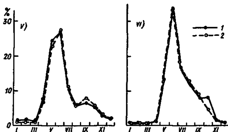
Рис. 3. Внутригодовое распределение водных ресурсов территорий экономических регионов СССР (в % от годовых водных ресурсов).
