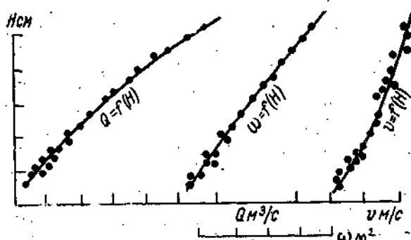
Рис. 17. Кривая расходов воды
