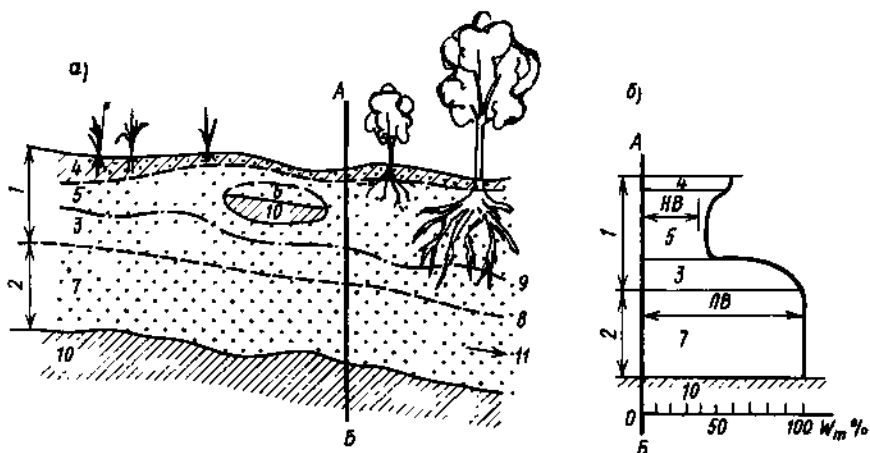
Рис. 5.2. Схема залегания вод зоны аэрации и грунтовых вод а) и вертикального распределения влажности грунта по разрезу А — Б после обильного увлажнения б): зоны: 1 — аэрации, 2 — насыщения, 3 — капиллярные, 4 — почвенные подвешенные воды, 5 — инфильтрующиеся воды зоны аэрации, 6 — верховодка, 7 — грунтовые воды, 8 — поверхность (зеркало) грунтовых вод, 9 — поверхность капиллярной зоны («капиллярной каймы»), 10 — водоупорный пласт, 11 — направление потока грунтовых вод, НВ — наименьшая влагоемкость, ПВ — полная влагоемкость
