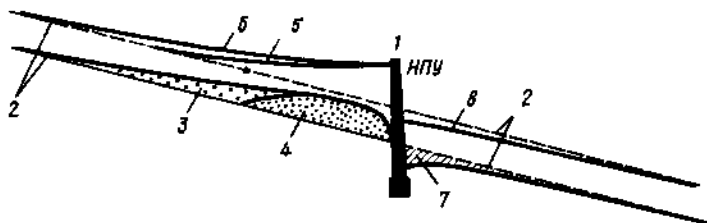
Рис. 6.23. Схема заиления и занесения верхнего бьефа и размыва нижнего бьефа гидроузла:
