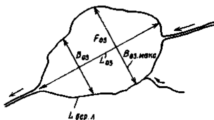
Рис. 7.2. Морфометрические характеристики озера
