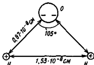
Рис. 1.1. Строение молекулы воды
