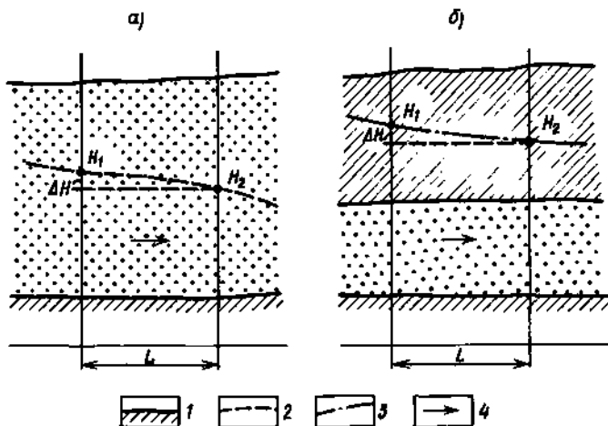
Рис. 5.5. Схема движения подземных вод в зоне насыщения (а — безнапорные грунтовые воды, б — напорные артезианские воды): 1 — водоупорный пласт, 2 — уровень грунтовых вод (кривая депрессии), 3 — линии пьезометрического напора (пьезометрическая кривая), 4 — направление движения подземных вод
