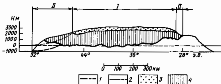
Рис. 4.2. Поперечный разрез Гренландского ледникового покрова (по Б. Фриструпу). Обозначения см. на рис. 4.3. Пунктир — профиль выводного ледника
