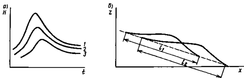
Рис. 6.17 Схема трансформации паводочной волны: а — график изменения уровня воды в трех створах, расположенных последовательно вдоль русла; б — продольные профили паводочной волны и ее длины в два последовательных момента времени
