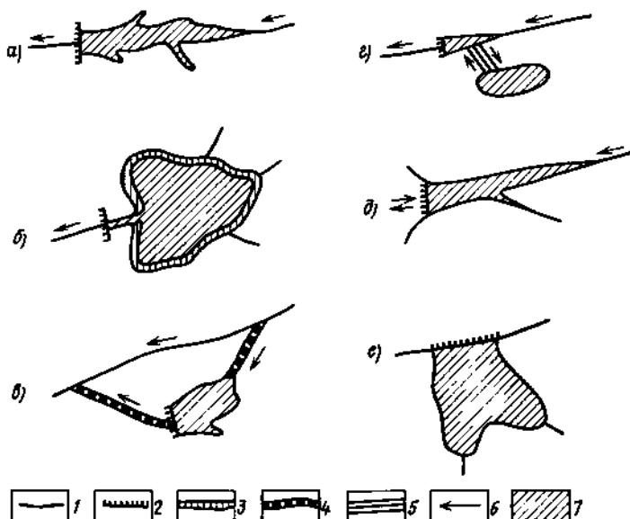
Рис. 8.1. Основные типы водохранилищ: а — долинное запрудное, б — котловинное запрудное (подпруженное озеро), в — котловинное наливное, г — котловинное наливное при гидроаккумулирующей электростанции, д — долинное запрудное в эстуарии при приливной электростанции, е — котловинное запрудное в опресненном морском заливе, 1 — река, 2 — плотина, 3 — затопленная при подпоре береговая зона озера, 4 — подводящий и отводящий каналы, 5 — водоводы, 6 — направление течения, 7 — зеркало водохранилища
