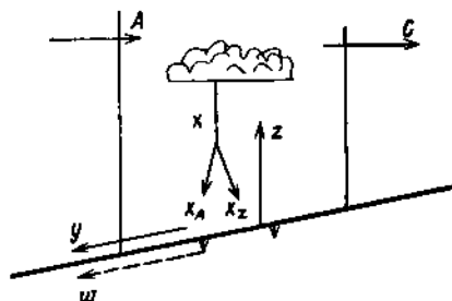
Рис. 3.3. Схема внутриматерикового влагооборота
