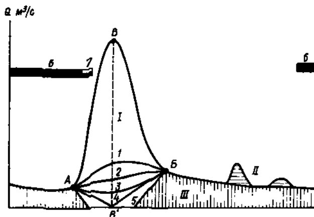
Рис. 6.10. Схема расчленения гидрографа реки по видам питания: питание: I — снеговое, II — дождевое, III — подземное; A, B и B' — начало, конец и пик половодья; 1—5 — линии, разделяющие снеговое и подземное питание в период половодья при различном характере взаимодействия речных и грунтовых вод (пояснение см. в тексте). 6 — ледостав, 7 — ледоход
