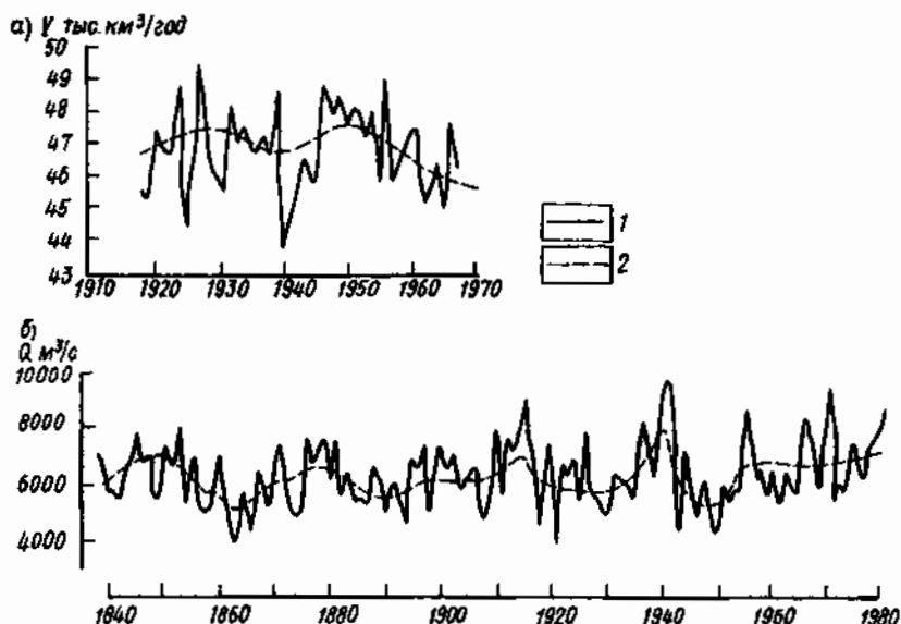
Рис. 6.7 Изменения суммарного стока рек земного шара, по Р. К. Клинге, а и стока Дуная б: 1 — средние годовые величины стока, 2 — осредненные (сглаженные) значения стока
