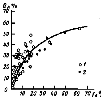
Рис. 4.6. Зависимость доли ледниковой составляющей годового стока ( Q_{\text{л}}\% ) от относительной площади оледенения бассейна (п. Г. Н. Голубеву): 1 — Средняя Азия, 2 — Кавказ
