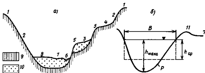
Рис. 6.3. Поперечный профиль долины а и русла реки б:
