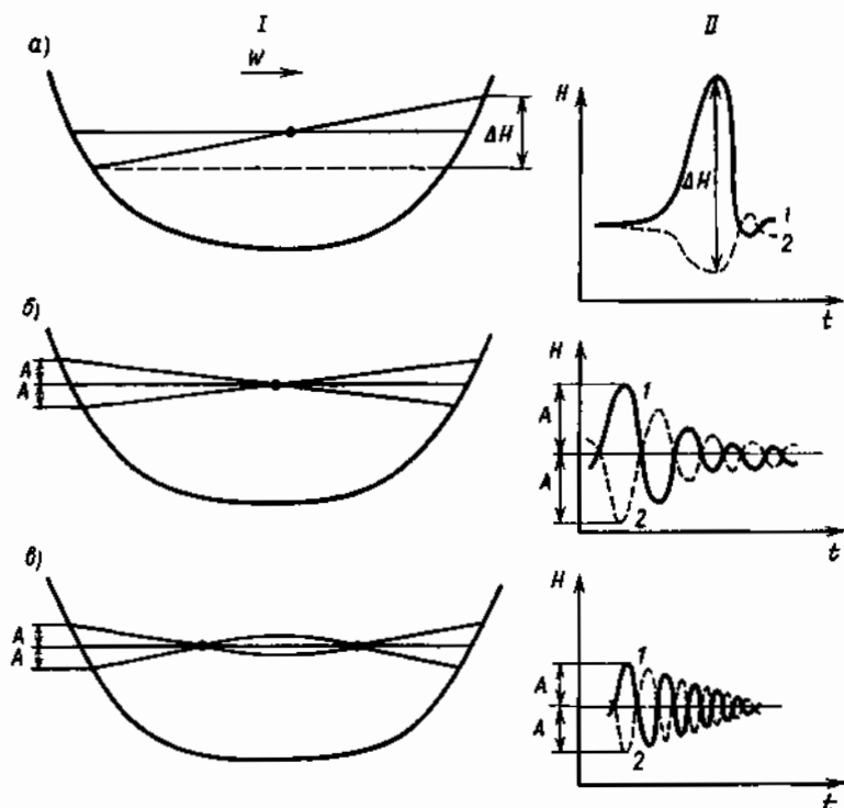
Рис. 7.7. Схема депрессии уровня озера при сплошно-нагонных явлениях (а), одноузловой (б) и двухузловой (в) сейсмах: I — поперечный разрез, II — колебания уровня у противоположных берегов (1,2) озера
