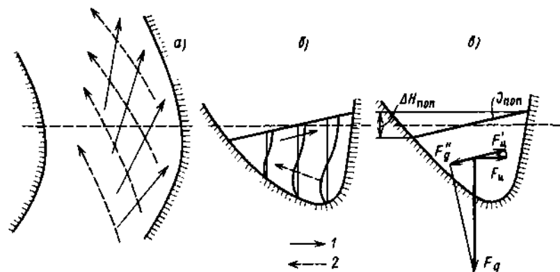
Рис. 6.16. Схема поперечной циркуляции на изгибе речного потока в плане а и поперечном разрезе б и схема действующих сил в: 1 — поверхностные струи, 2 — придонные струи
