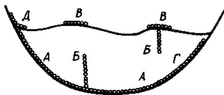
Рис. 4.4. Схема поперечного строения ледника: алекомые морены: А — придонная, Б — внутренняя, В — срединная, Г — поперечная, Д — боковая
