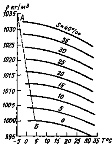
Рис. 1.5. Зависимость плотности воды при нормальном атмосферном давлении от температуры и солености. AB — линия наибольшей плотности
