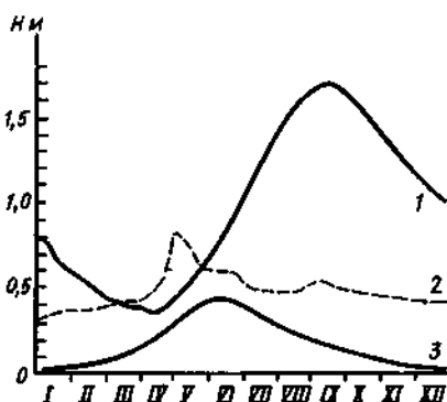
Рис. 7.6. Типичные графики сезонных колебаний уровня озер: Телецкого (1), Плещеева (2), Ладожского (3)
