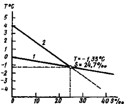
Рис. 1.4. Зависимость температуры замерзания T_{\text{зам}} 1 и температуры наибольшей плотности T_{\text{плот.пл}} 2 от концентрации S (график Хелланд-Хансена)
