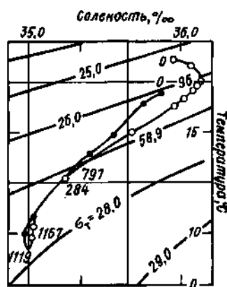
Рис. 10.23. Пример T, S -кривых для двух станций НИС «Атлантик», 1932 г. Цифрами (м) помечены некоторые горизонты
