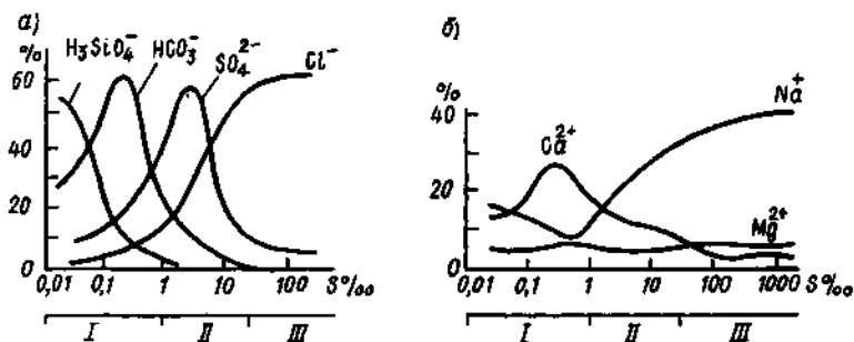
Рис. 1.2. Зависимость содержания главных анионов а и катионов б в солевом составе природных вод (в %) от минерализации (солёности) воды по М. Г. Валяшко:
