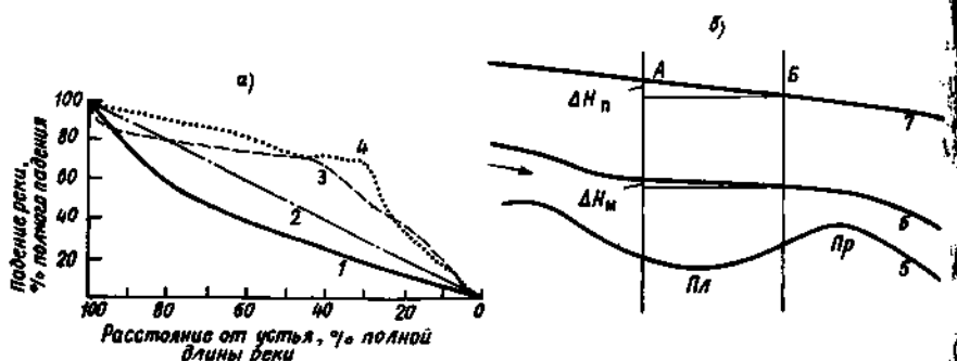
Рис. 6.5. Продольные профили реки a и ее участка б :
