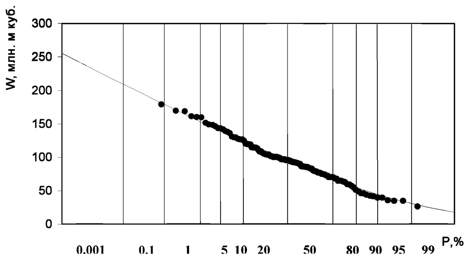
Рис.3 Эмпирическое распределение годовых объемов притока к озерам Песьво и Удомля и его аппроксимация аналитическим распределением С.Н.Крицкого и М.Ф.Менкеля с параметрами: W_{ср}=95.0 млн. м 3 ; C_v=0.34 ; C_s/C_v=1.0 .
