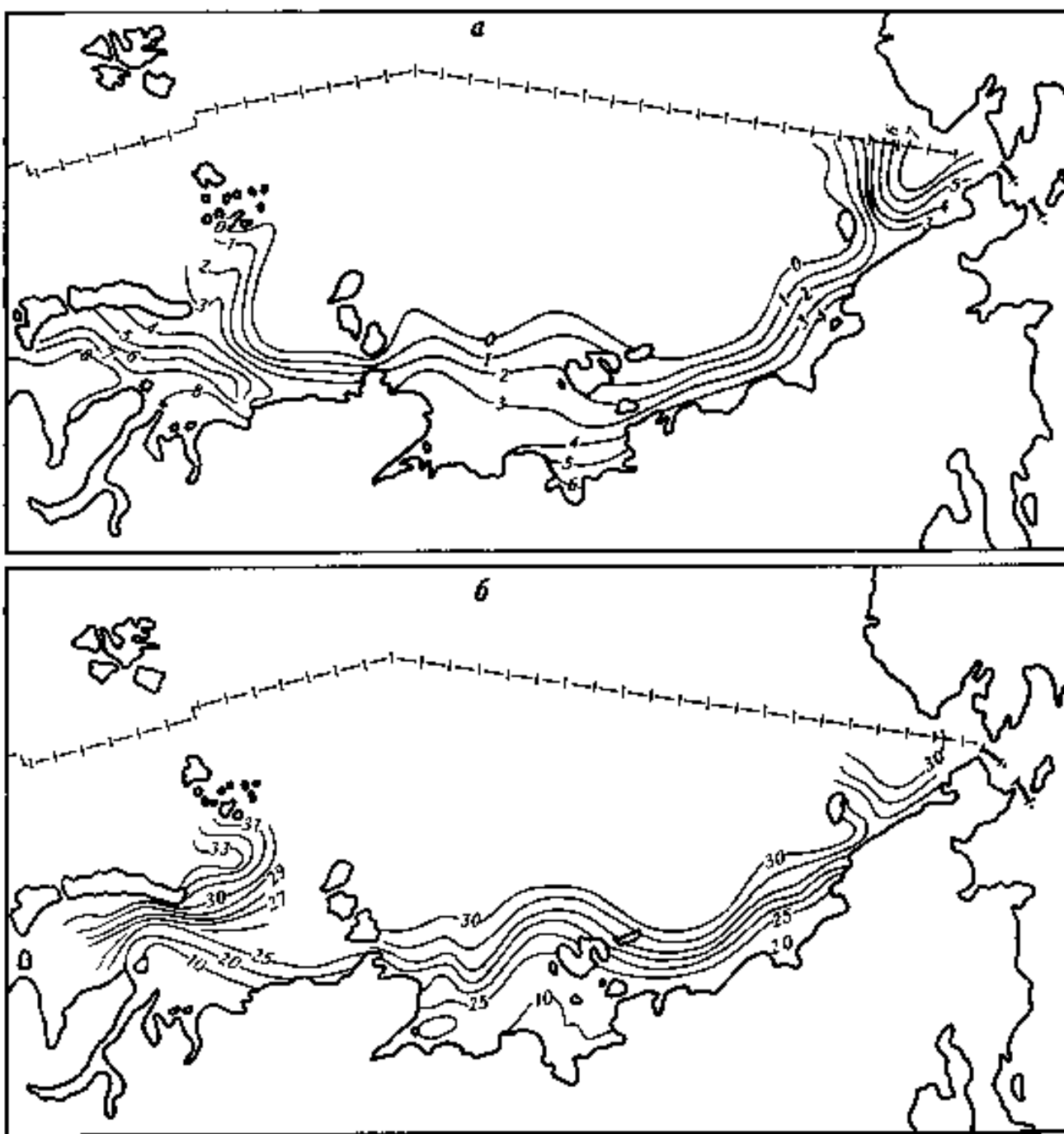
Рис. 26. Распределение температуры (а) и солёности (б) на поверхности арктических морей летом
