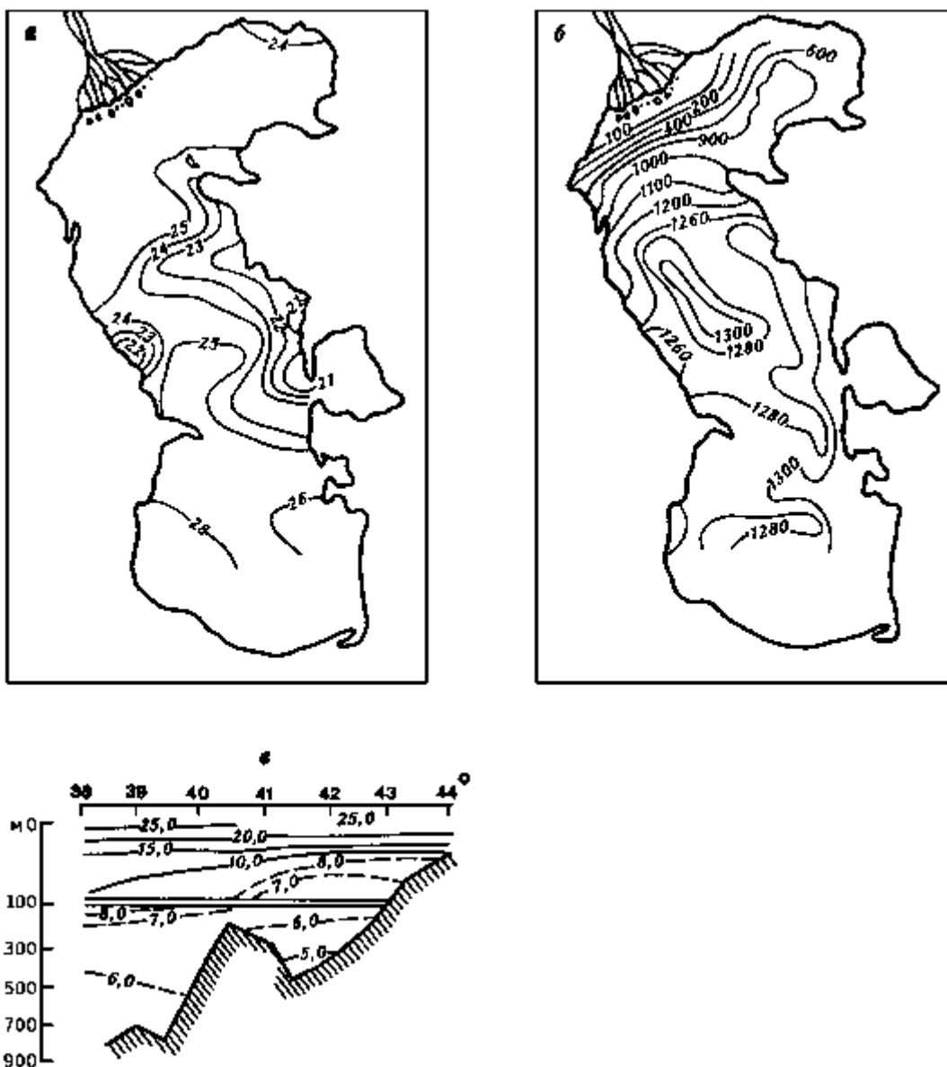
Рис. 5. Распределение температуры (а) и солёности (б) на поверхности и температуры на разрезе по меридиану 51° в. д. (в) в Каспийском море летом
