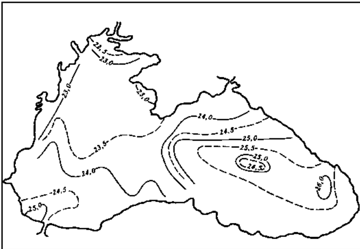
Рис. 10. Распределение температуры воды на поверхности Черного моря летом
