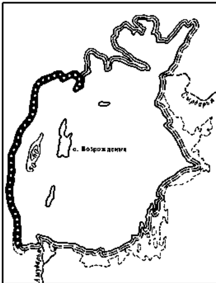
Рис. 2. Типы берегов и рельеф дна Аральского моря. Усл. обозначения см. рис. 1.
