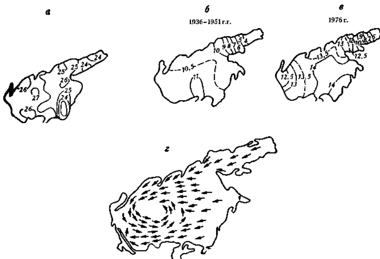
Рис. 9. Распределение температуры (а), солёности воды на поверхности моря за 1936—1951 гг. (б), в 1976 г. (в) и результирующие поверхностные течения (г)
