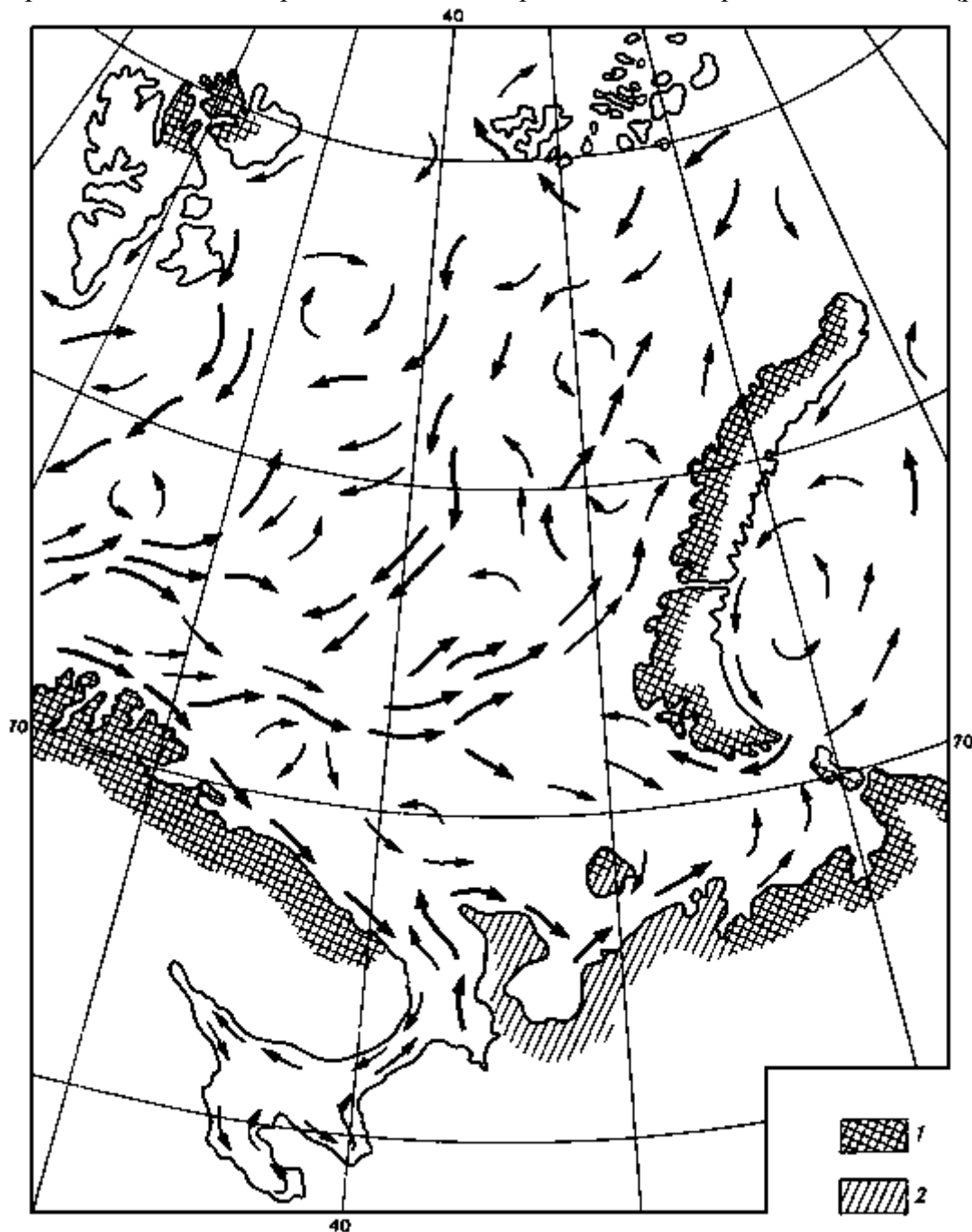
Рис. 32. Течения на поверхности и характер приливов в Баренцевом море: 1 — приливы полусуточные; 2 — приливы полусуточные мелководные
