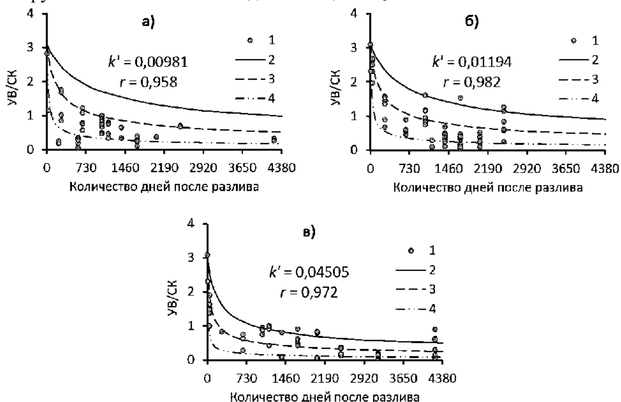
Рисунок 2 –Изменение соотношения VB/CK в составе нефтяных сликов с течением времени на черноморском побережье в районе г. Новороссийска (а), черноморском (б) и азовском (в) побережьях Керченского пролива: 1 – пробы сликов, 2–4 – кривые, аппроксимирующие трансформацию сликов толщиной 30 мм (2) и 3 мм (3, 4) в средней (2, 3) и верхней (4) частях литоральной зоны
