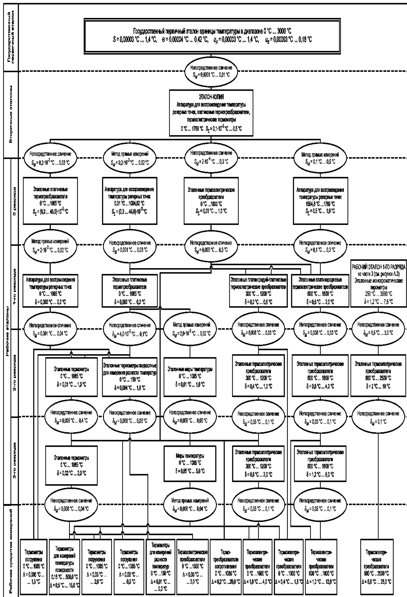
Рисунок А.2 – Поверхная схема для контактных термометров в диапазоне 0 °C ... 3000 °C
