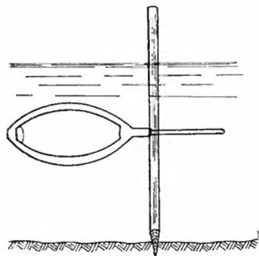
Батометр-тахиметр Глушкова.
