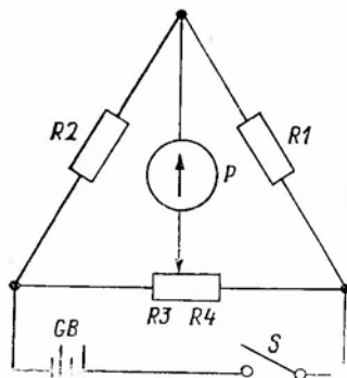
Принципиальная схема электротермометра.
