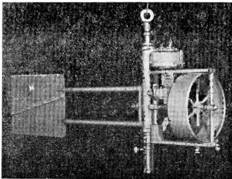
Морская вертушка.
