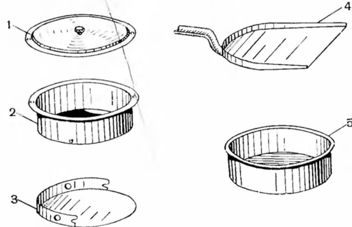
Снеговой испаритель ГГИ-500-6.
