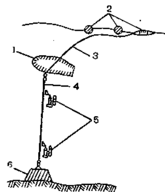
Схема буйковой станции.
