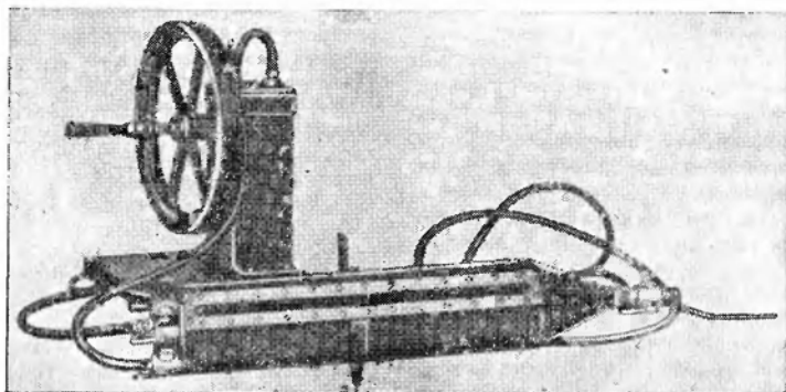
Батометр вакуумный.
