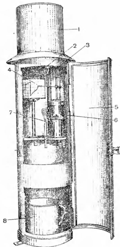
Общий вид пловниграфа с принудительным сливом.
