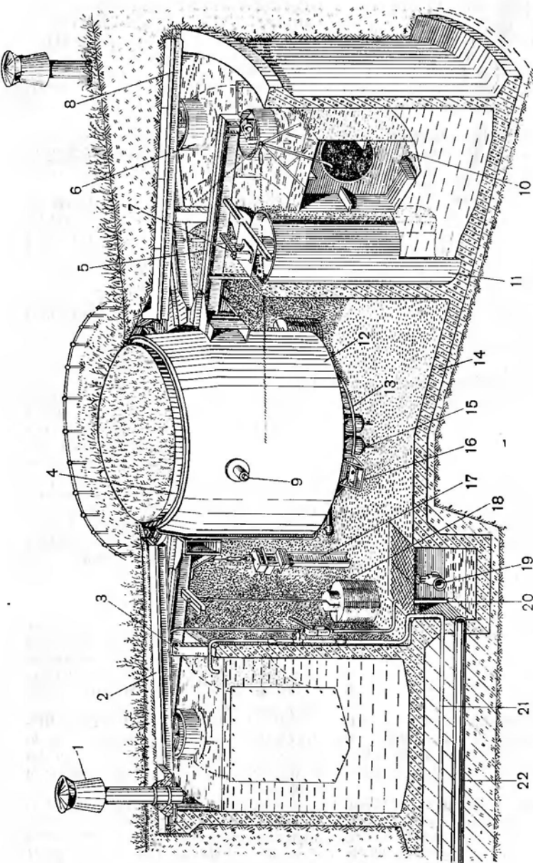
Вертикальный разрез гидравлического испарителя.
