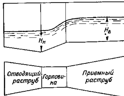
Схема гидрометрического лотка.
