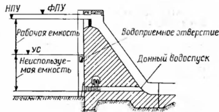
Характерные элементы водохранилища.
