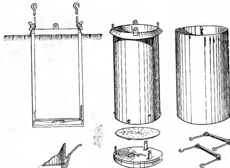
Весовой почвенный испаритель ГГИ-500-50.
