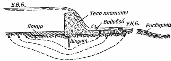
Флютбет водосливной плотины.
