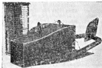
Батометр-ловушка Шамова.
