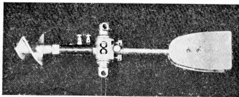
Гидрометрическая вертушка ГР-55 (внешний вид).
