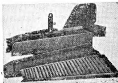
Батометр-ловушка «Дон».
