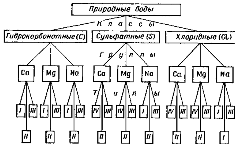
Схема классификации природных вод по преобладающему аниону и соотношению между главнейшими катионами (по О. А. Алекину).
