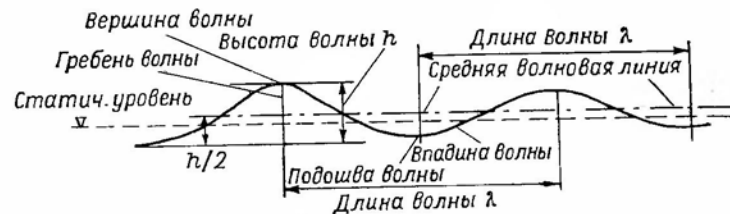
Профиль ветровой волны.
