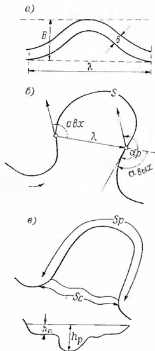
Типы меандрирования.
