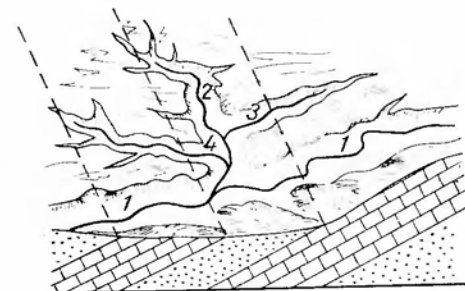
Схема расположения рек относительно простираания пластов горных пород. 1 — консеквентные, 2 — субсеквентные, 3 — ресекувентные, 4 — обсеквентные реки.
