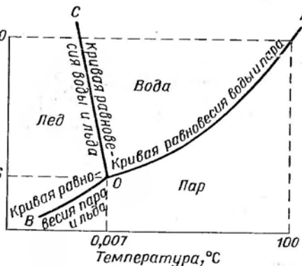
Диаграмма состояния воды.
