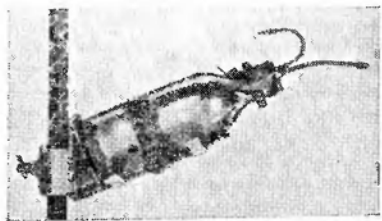
Батометр-бутылка ГИИ с креплением на штанге.
