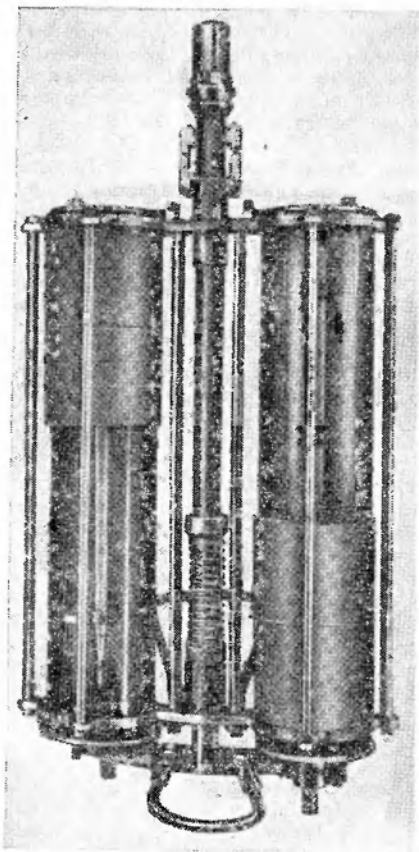
Батометр Молчанова.
