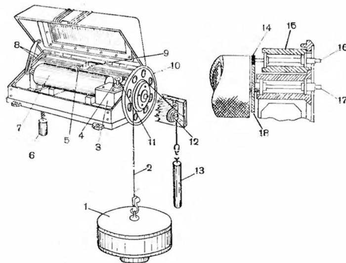
Самописец уровня воды «Валдай».
