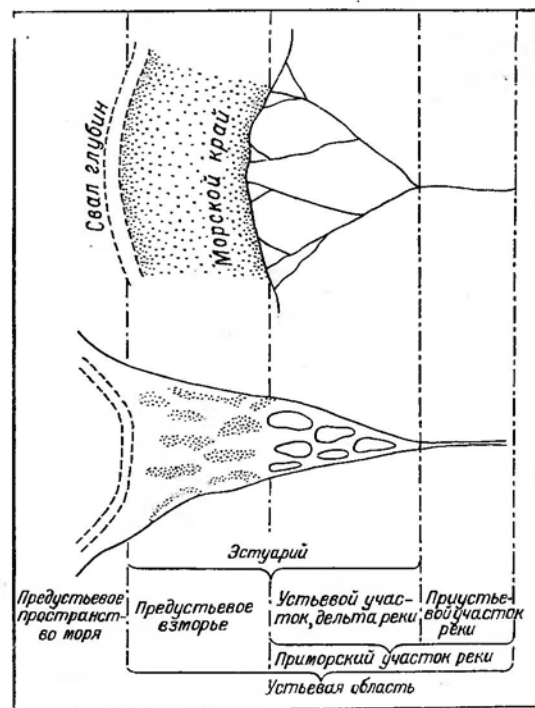
Схематизированные типы устьев рек.
