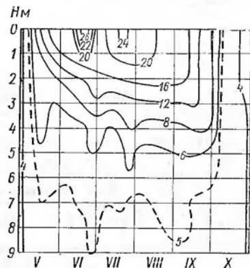
Термоизоплеты.
