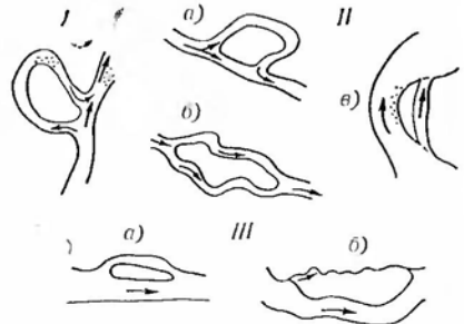
Пойменные острова (по И. В. Попову).
