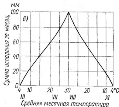
Графики Майера. а — испарение с поверхности воды, снега и льда, б — испарение с почвы, в — для расчета испарения с растительного покрова (транспирация).
