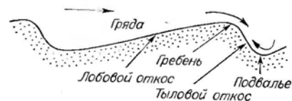
Продольный профиль песчаной гряды.
