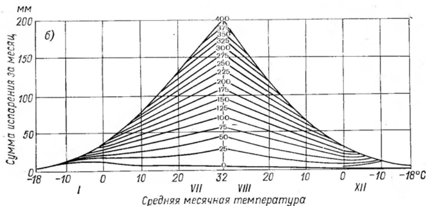
Графики Майера. а — испарение с поверхности воды, снега и льда, б — испарение с почвы, в — для расчета испарения с растительного покрова (транспирация).
