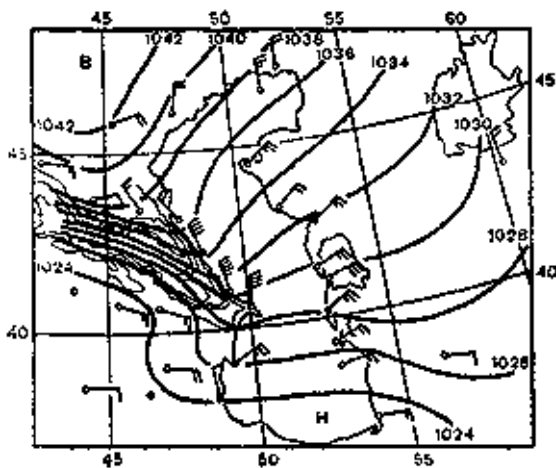
Синопогическая ситуация при развитии Бакинского норда.
