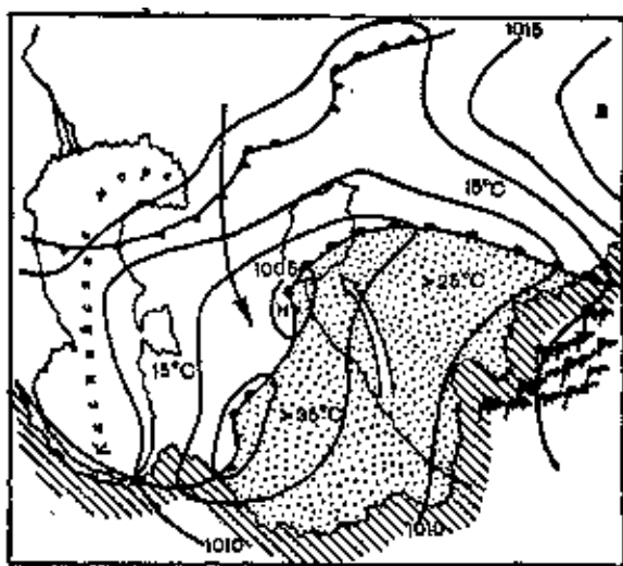
Синоптическая ситуация при развитии Гармсиля в Средней Азии.
