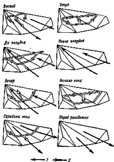
Схема развития Горно долинных (1) и Склоновых (2) ветров
