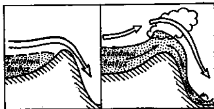
Схема накопления холодного воздуха на наветренной стороне горного хребта (слева) и обвал его на подветренном склоне (справа) при Боре.
