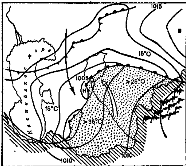
Синоптическая ситуация при развитии Гармсилы в Средней Азии.
