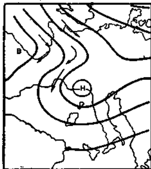
Схема приземного барического поля при возникновении Мистрала в тылу генуэзского циклона.
