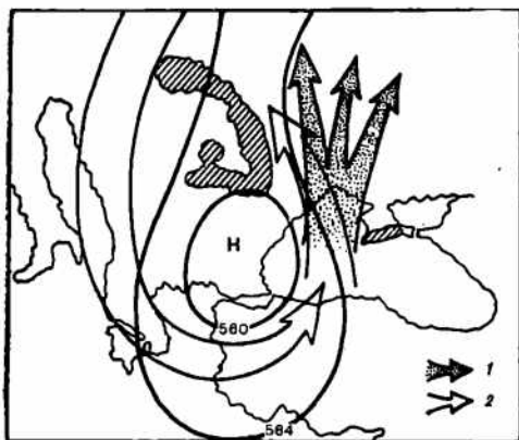
Схема приземных воздушных потоков и изогипсы поверхности 500 гПа при всаниковении Смерчей на Украине.
