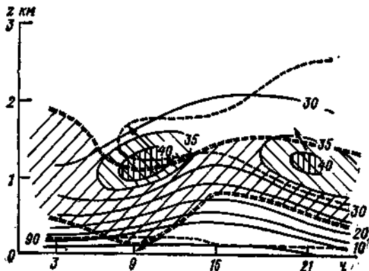
Изоахы (м/с) на вертикально-временном разрезе при развитии над Киевом 5 января 1969 г. сильно восточной Мезоструи со скоростью ветра на ее оси (высота 1 км) более 40 м/с.
