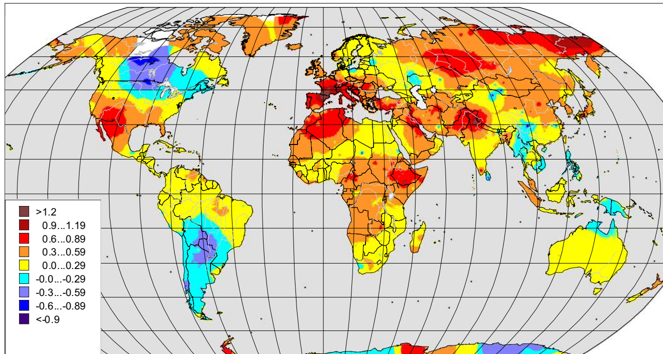
Рис. 1.12. Тренды среднемесячной температуры воздуха за 1976–2010 гг. ( ^{\circ}\text{C}/10 лет). Май
