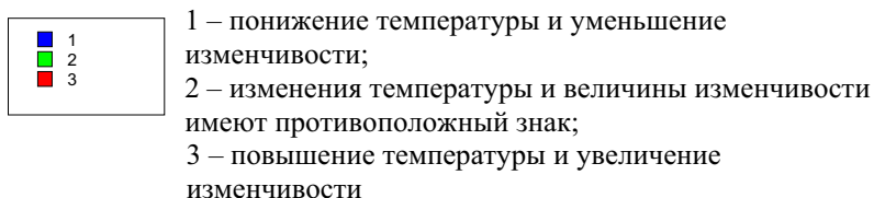
Рис. 1.35. Соотношение изменений климата и его изменчивости. Январь
