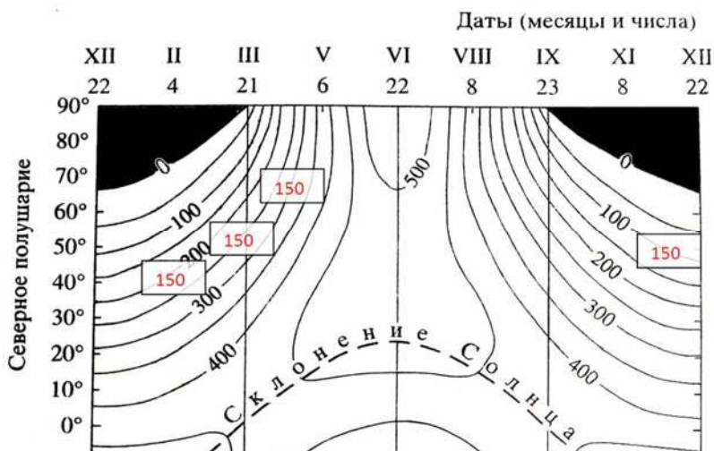
Рис. 4.5. Прямая солнечная радиация на верхней границе атмосферы ( \text{Вт/м}^2 ) и широты с положительными трендами: 45–55 °с.ш. (зима), 55–60 °с.ш. (зима–весна), 65–70 °с.ш. (конец весны), 45–50 °с.ш. (осень)
