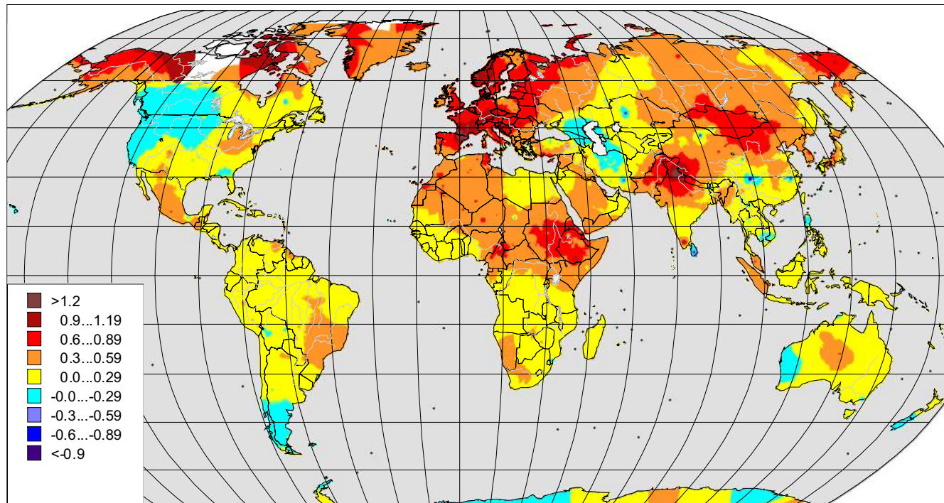
Рис. 1.11. Тренды среднемесячной температуры воздуха за 1976–2010 гг. ( ^{\circ}\text{C}/10 лет). Апрель
