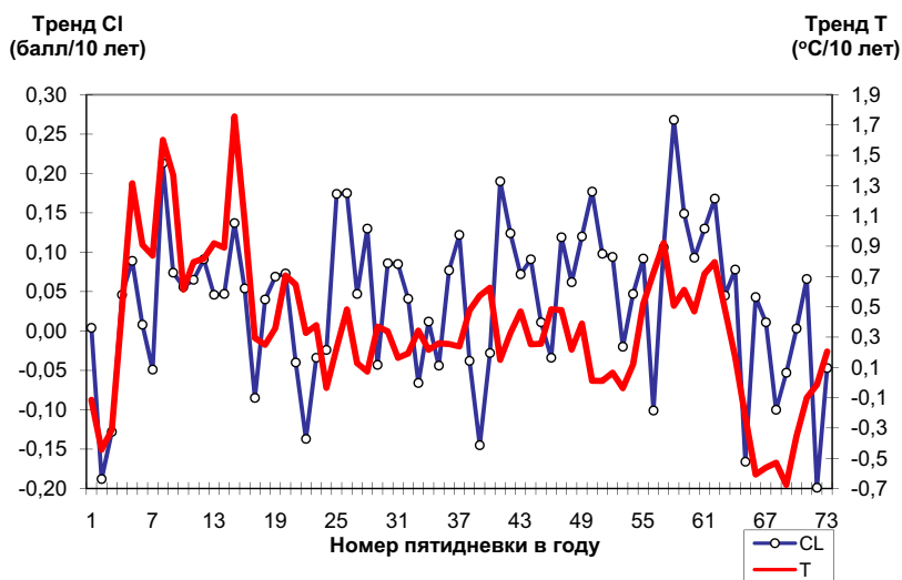
Рис. 4.6. Тренды температуры воздуха (T) и количества общей облачности (CL) по пятидневкам года
