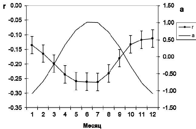
Рис. 3.34. Северо-южное ускорение (а) движения Земли и радиус-вектор (r) полюса Земли за 1920–1954 гг.
