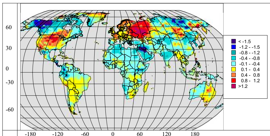
Рис. 1.28. Тренды временной изменчивости за 1974–2005 гг. (°C/10 лет). Ноябрь
