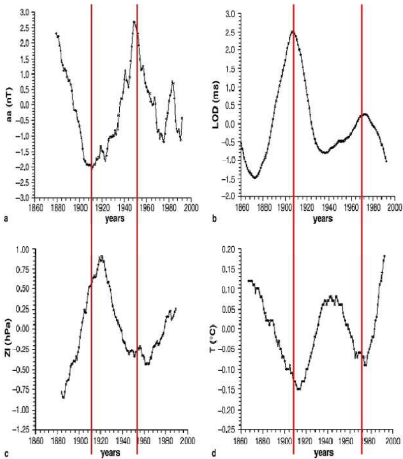
Рис. 1.5. Отклонения от тренда среднегодовых значений после сглаживания по 23 годам: а) индекс геомагнитной активности aa ; б) продолжительность суток LOD; в) индекс зональной циркуляции Северного полушария ZI; д) аномалии температуры воздуха Северного полушария. Рис. из [107]
