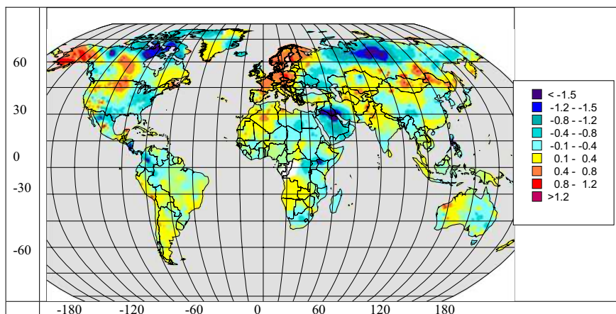
Рис. 1.27. Тренды временной изменчивости за 1974–2005 гг. (°C/10 лет). Октябрь
