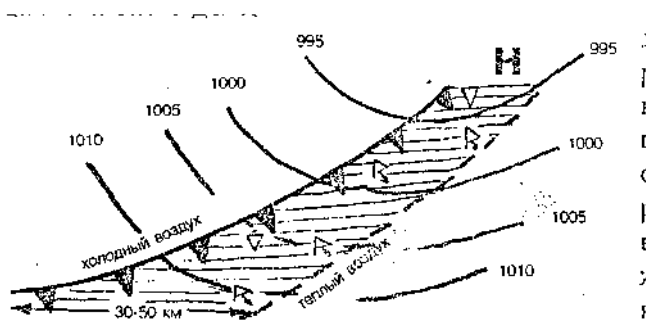
Рис. 29 Расположение грозы на холодном фронте
