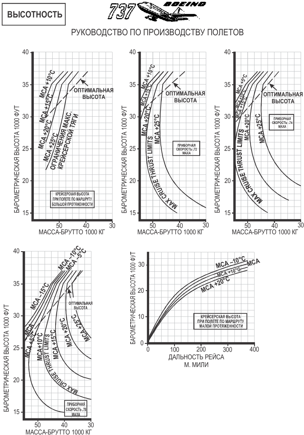
Рис. А6-3. Оптимальный эшелон полета (для В-737) в зависимости от взлетной массы и отклонения температуры от стандартной
