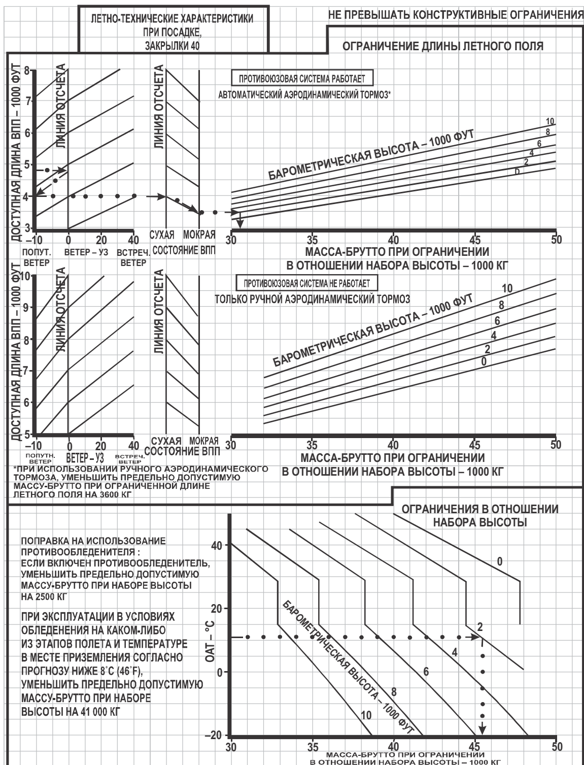
Рис. А6-6. Расчет посадочных характеристик
