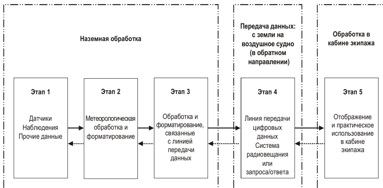
Рис. А8-1. Схема системы METLINK
