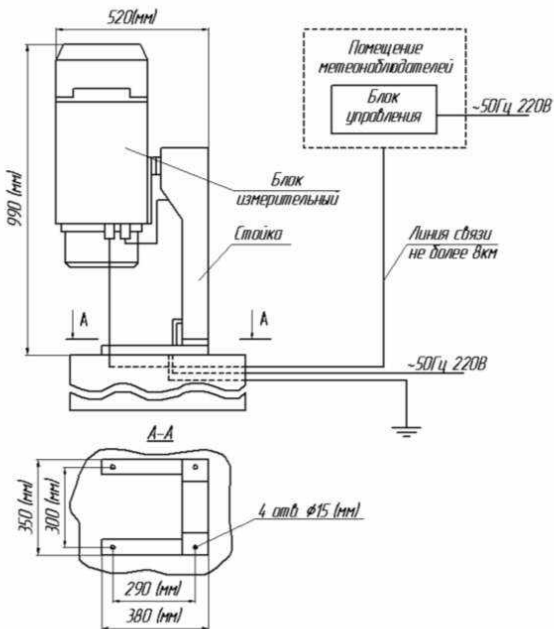
Рисунок А.5 – Схема сборки ДОЛ-2
