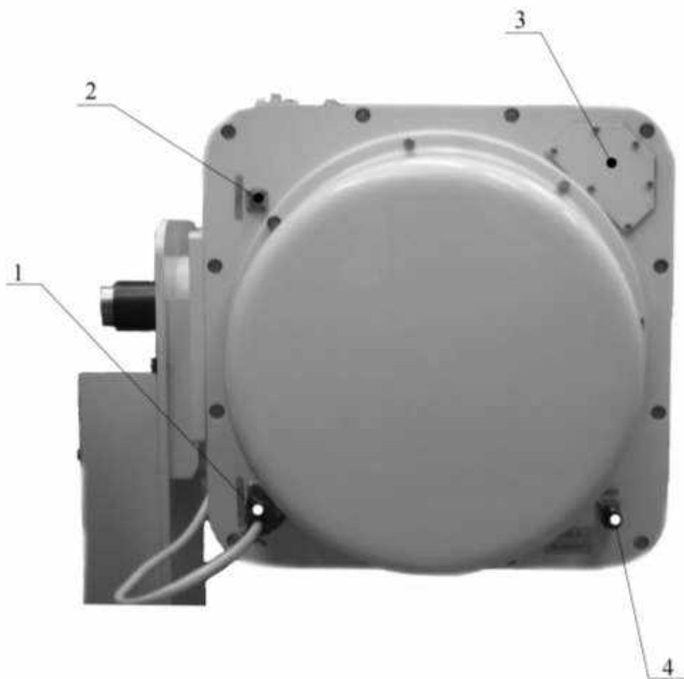
Рисунок А.4 – Блок измерительный вид снизу
