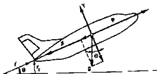
Рис. 3.2. Схема сил, действующих на самолет при подъеме.
