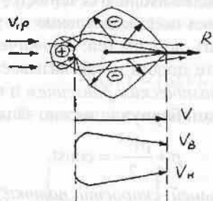
Рис. 1.3. Обтекание крыла потоком при \alpha = 0 .
