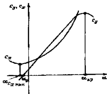
Рис. 1.5. Зависимость коэффициентов c_y и c_x от угла атаки \alpha .
