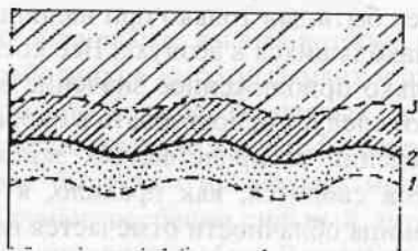
Рис. 9.18. Схема структуры нижней границы облаков:
