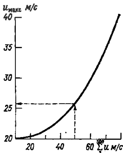
Рис. 7.8. Определение максимальной скорости ветра при шквале.
