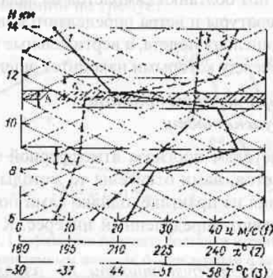
Рис. 8.7. Графический метод прогноза болтанки самолетов.
