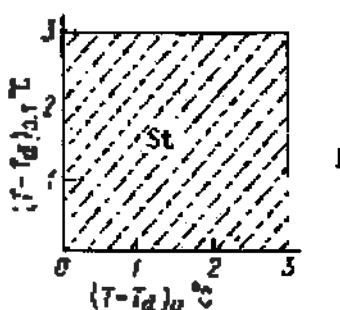
Рис. 9.17. График для прогноза облачности ниже 300 м, используемый в аэропорту Черский.
