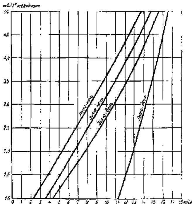
Рис. 7.5. График зависимости скорости ветра от горизонтального градиента давления.
