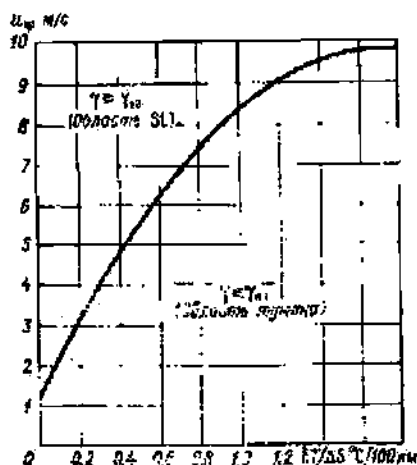
Рис. 9.21. График для прогноза адвективного тумана (по И.В. Кошеленко).
