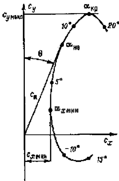
Рис. 1.6. Поляра крыла самолета.
