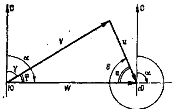
Рис. 7.1. Навигационный треугольник скоростей.
