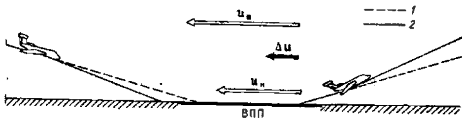
Рис. 7.3. Пример влияния вертикального сдвига ветра на взлет и посадку: 1 – предполагаемая, 2 – действительная траектория движения ВС.
