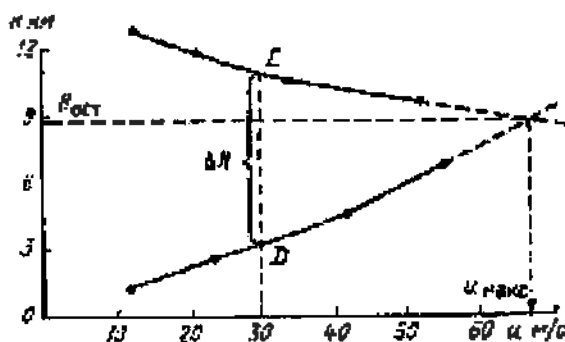
Рис. 7.17. Определение параметров струйного течения (по методу Е. Рейтера).
