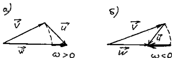
Рис. 7.2. К определению эквивалентного ветра: a - \omega > 0 , b - \omega < 0 .
