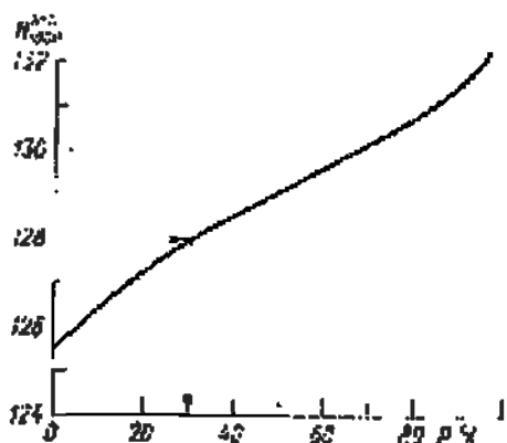
Рис. 10.2. График для определения вероятности возникновения гололеда.
