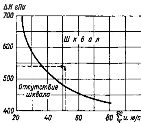
Рис. 7.7. График для определения возможности шквала.
