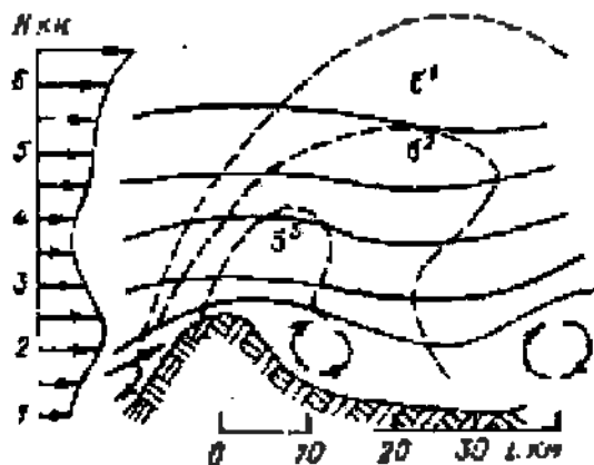
Рис. 8.5. Характеристика турбулентных зон над горами. 6 1 – слабая, 6 2 – умеренная, 6 3 – сильная болтанка.
