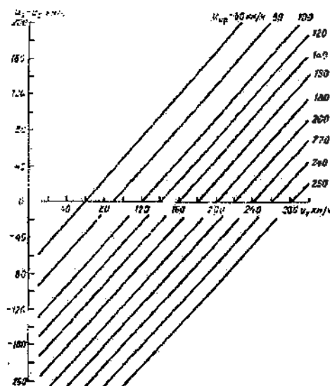
Рис. 7.16. Номограмма для прогноза скорости ветра на высотах на 24 ч (по методу Э.С. Ильиной).
