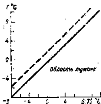
Рис. 9.23. График для прогноза адвективного тумана (по методу А.А. Шадриной).
