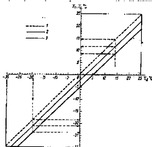
Рис. 9.19. График для прогноза радиационного тумана по методу Н.В. Петренко: 1 – линия дымки, 2 – линия слабого тумана, 3 – линия сильного тумана.
