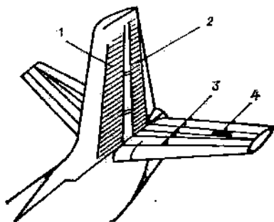
Рис. 2.1. Общий вид оперения самолета: 1 – киль, 2 – руль направления, 3 – стабилизатор, 4 – руль высоты.
