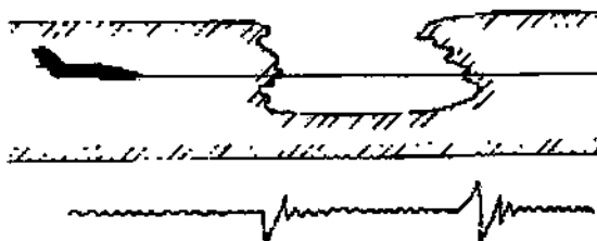
Рис. 8.3. Вид записи акселерографа при полете ВС вблизи «стен» облаков.
