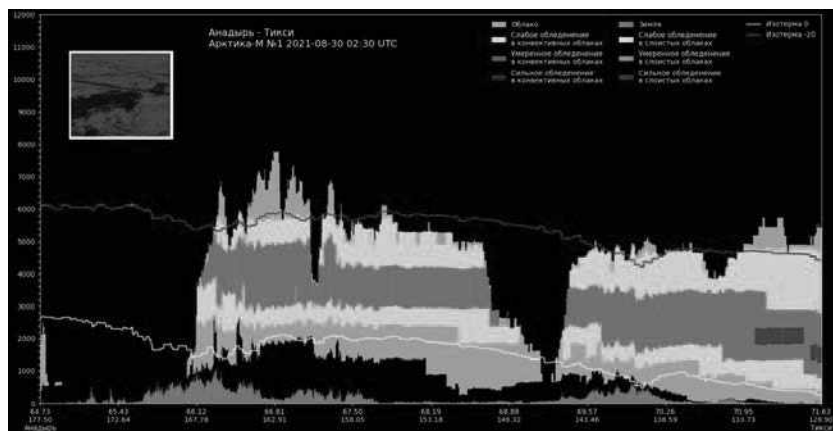
Рисунок 5.2 - Вертикальные разрезы облачности и обледенения по трассе Анадырь – Тикси по данным КА «Арктика-М» №1
