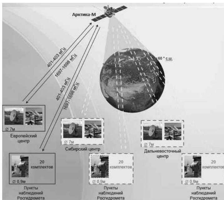
Рисунок 5.1 - Космическая система двухсторонней радиосвязи
