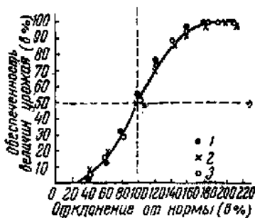
Рис. 15. Кривая обеспеченности различных величин урожая зерновых культур и показателя увлажнения за год, выраженные в процентах от нормы (средне многолетней величины) для полусасушливой зоны:
