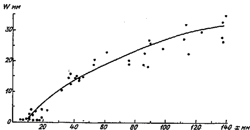
Рис. 18. Зависимость запасов продуктивной влаги в слое почвы 0–20 см ( W ) по непаровым предшественникам, подготовленной для посева озимой пшеницы, от суммы осадков за предпосевной месяц ( x ).
