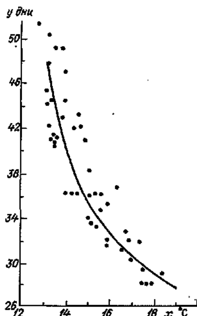
Рис. 27. Зависимость продолжительности межфазного периода от выхода в трубку до колошения озимой пшеницы ( y ) от уровня температуры воздуха за этот период ( x ).
