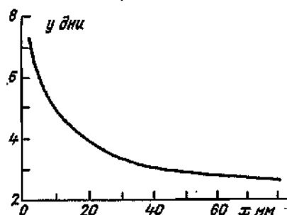
Рис. 22. Зависимость продолжительности периода посев — массовое прорастание семян озимой пшеницы ( y ) от количества эффективных осадков за месяц до начала посева ( x ).
