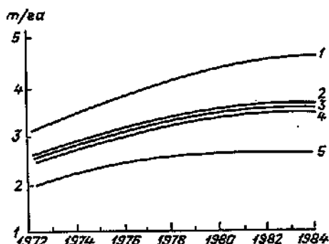
Рис. 5. Урожайность (т/га) по тренду озимой пшеницы по разным предшественникам (1-5) в совхозе „Гигант“ Сальского района Ростовской области в 1972-1984 гг.
