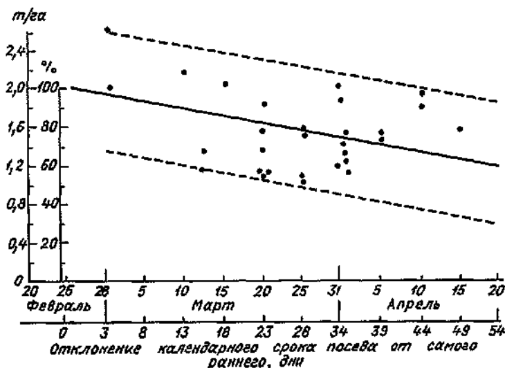
Рис. 7. Снижение урожайности (т/га, %) ярового ячменя в зависимости от отклонения (дни) календарного срока посева от самого раннего. Ростовская область, 1958–1988 г.
