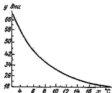
Рис. 23. Зависимость продолжительности периода посев — массовое кущение озимой пшеницы, возделываемой на черных парах или при орошении ( y ), от средней температуры воздуха за этот период ( x ).
