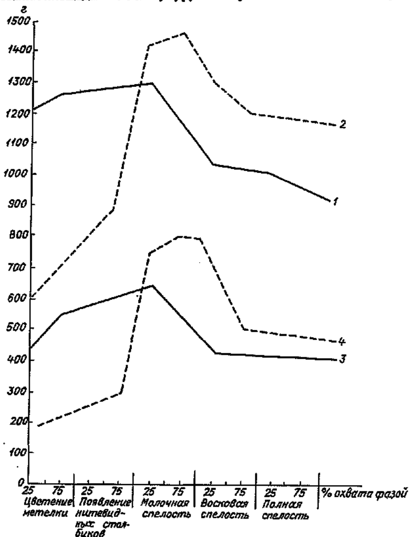
Рис. 15. Зависимость сырой и сухой массы (г) одного растения кукурузы от фазы ее развития (фаза, % охвата фазой) на агрометеорологической станции «Гигант» за 1987 и 1988 гг. 1 и 2 — сырая масса соответственно в 1987 и 1988 гг.; 3 и 4 — сухая масса соответственно в 1987 и 1988 гг.
