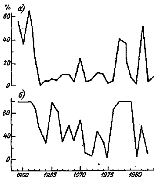
Рис. 4. Динамика формирования плоских и невозделанных озимых (% от всего посева в конкретном году) осенью (а) на фоне площади распространения (процент от общей площади посева) сильной засухи в сентябре (б) в Ростовской области за период 1959–1983 гг.
