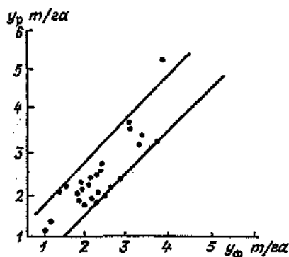
Рис. 31. Связь между расчетной урожайностью озимой пшеницы ( y_p ) по комплексной агрометеорологической оценке и фактической урожайностью ( y_ф ).
