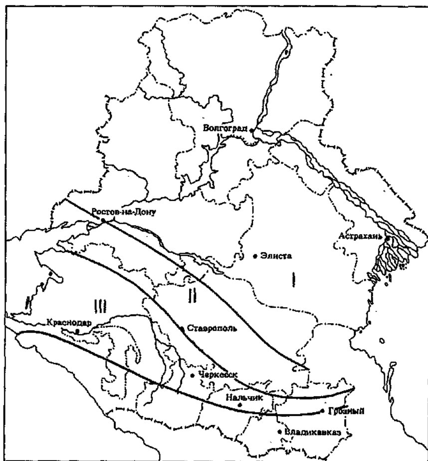
рис. 29. Районирование территории по разности в урожаях ярового и озимого ячменя. Зона I — у_{о.я.} > у_{я.я.} ; зона II — у_{о.я.} < у_{я.я.} .
