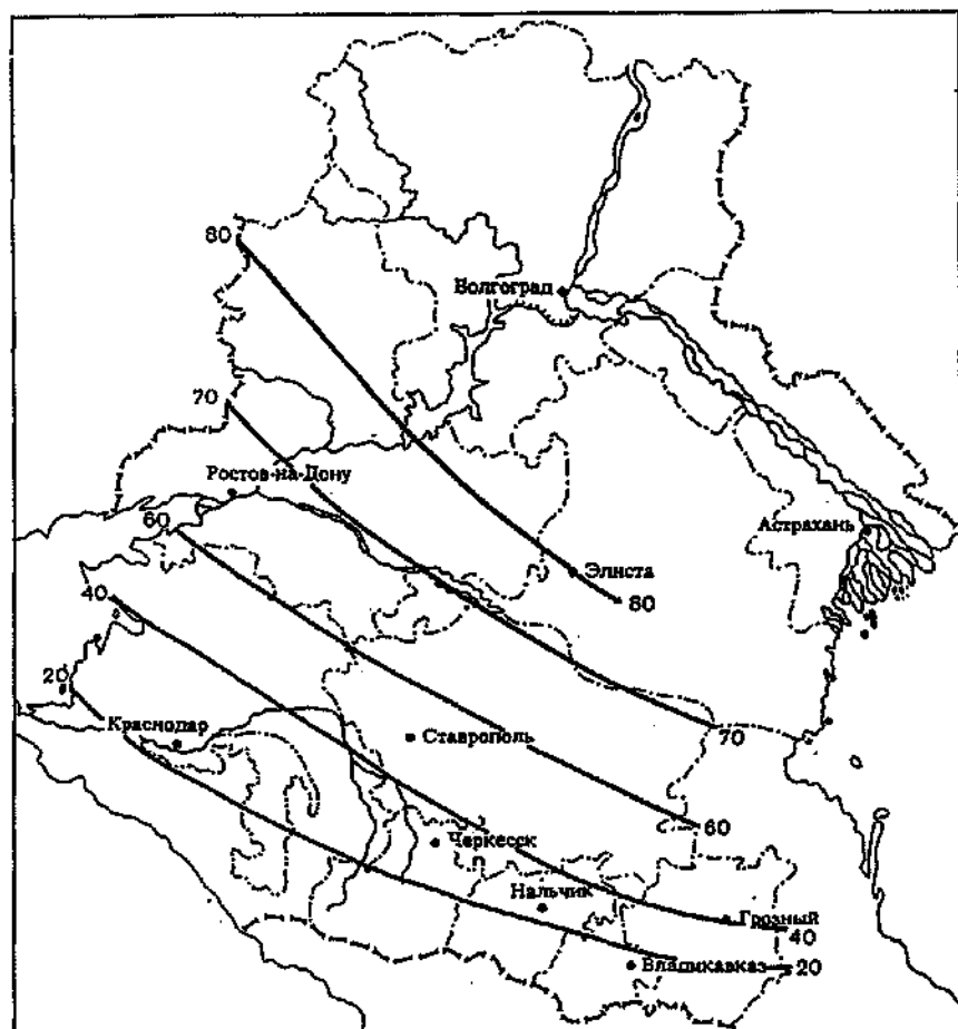
Рис. 28. Повторяемость (%) зим, в которые возможны значительные повреждения озимого ячменя.
