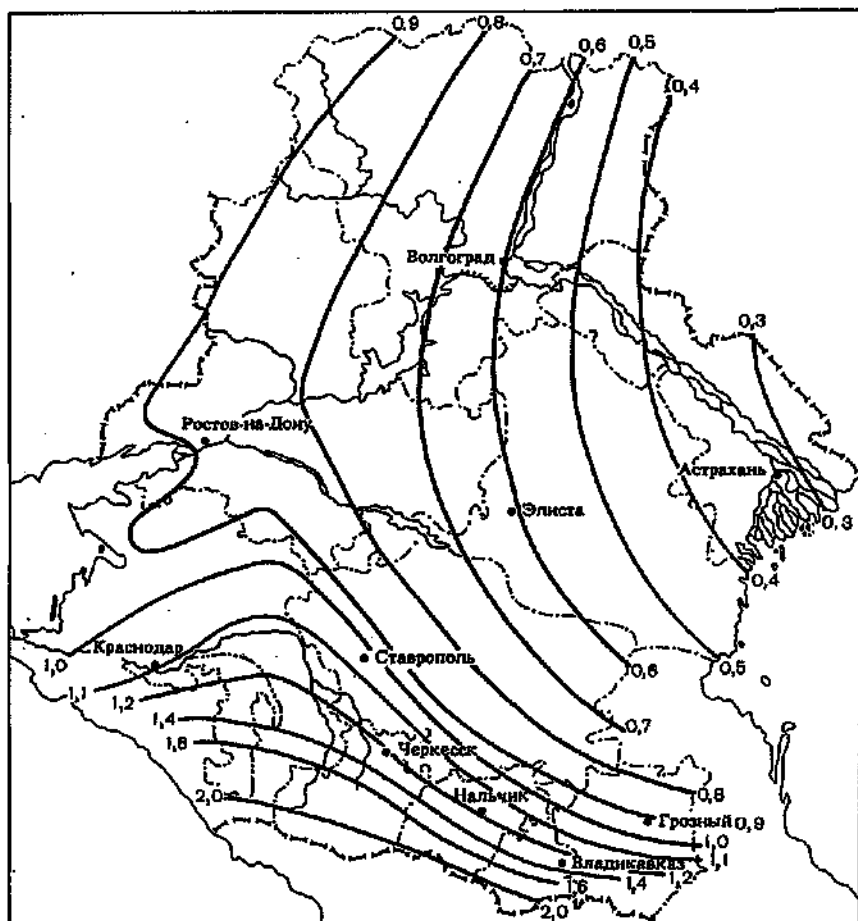
Рис. 1. Гидротермический коэффициент за вегетационный период (апрель—сентябрь, для Краснодарского края апрель—октябрь) на территории Северного Кавказа и низа Нижнего Поволжья в среднем за 1964—1988 гг.
