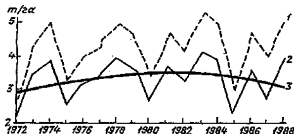
Рис. 6. Динамика урожайности (т/га) озимой пшеницы в совхозе „Гигант“ за 1972—1988 гг.
