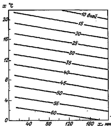
Рис. 24. Зависимость продолжительности (дня) периода посев — начало массового кушения озимой пшеницы, возделываемой по яровым предшественникам, от средней температуры воздуха за тот же период ( x ) и суммы эффективных осадков за месяц до посева ( x_1 ).
