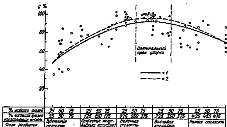
Рис. 16. Связь между накоплением сухой (1) и сырой (2) массы у (% от максимальной массы) и фазой развития кукурузы.
