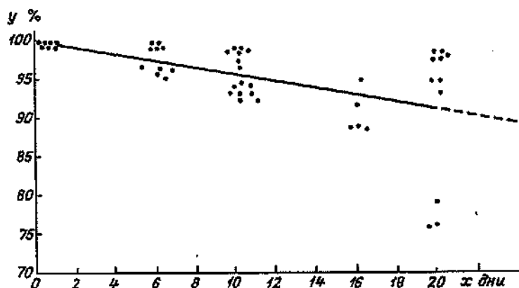
Рис. 11. Снижение урожайности подсолнечника (у) в зависимости от задержки сроков уборки (х).
