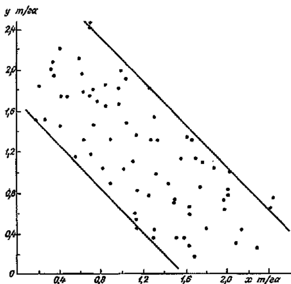
Рис. 14. Зависимость урожайности зерновых культур в Волгоградской области в текущем году ( y ) от их урожайности в прошлом году ( x ).
