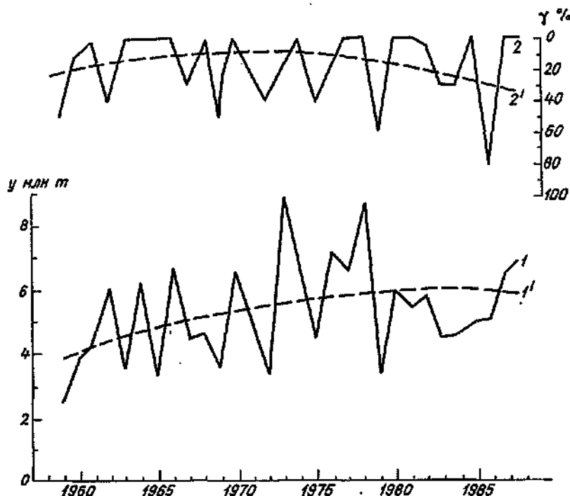
Рис. 2. Изменение валового сбора зерновых y(1) на фоне площади распространения сильной и очень сильной засухи y(2) в Ростовской области за период 1959—1988 гг.
