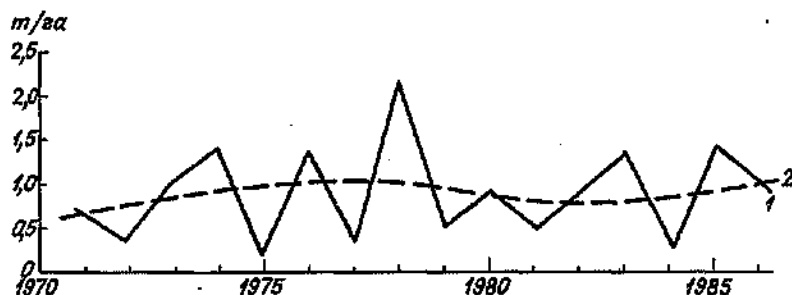
Рис. 13. Динамика урожайности (т/га) озимой ржи в сухостепной зоне каштановых почв (левобережье) Волгоградской области. 1 — урожайность; 2 — урожайность по тренду.
