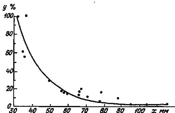
Рис. 20. Связь между количеством осадков, выпавших в предпосевной и послепосевной месяцы ( x ), и площадью плохих и незашедших осенью озимых по неурожаям предшественникам ( y ).
