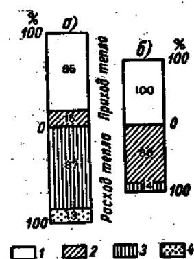
Рис. 94. Тепловой баланс.
