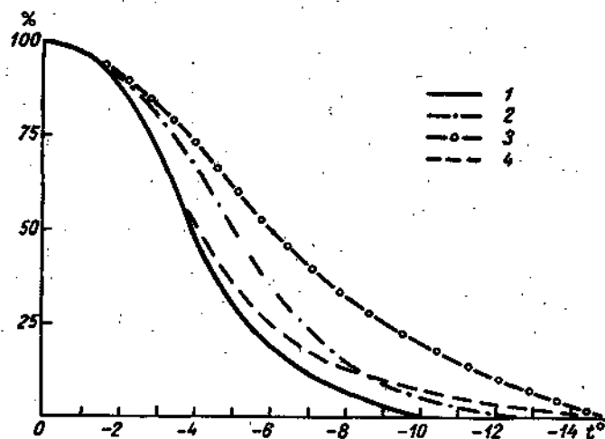
Рис. 31. Типы кривых вероятности наступления минимальных температур в разных местоположениях в субтропической зоне Западной Грузии.
