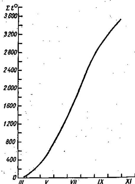
Рис. 4. Средние многолетние суммы активных температур выше 0^{\circ} нарастающим итогом (ст. Одесса).
