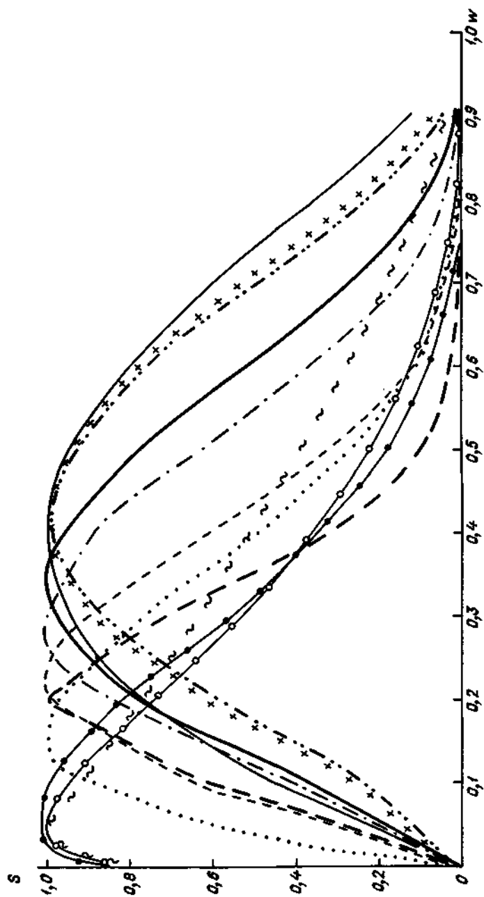
Рис. 126. Зависимость относительной продуктивности S от влагозапасов почвы в слое 0—50 см для твердых сортов яровой пшеницы по декадам вегетации. P_{0-50} = 25\% . Усл. обозначения см. рис. 11д.
