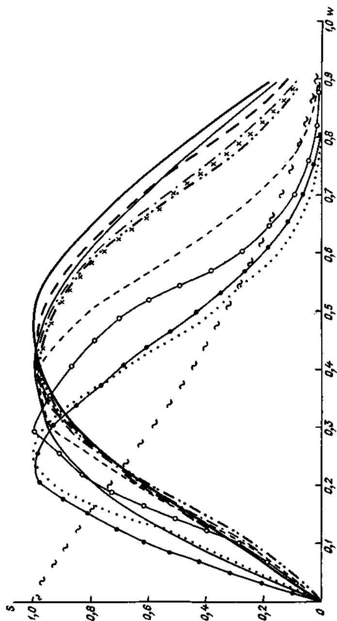
Рис. 12в. Зависимость относительной продуктивности S от влагозапасов почвы в слое 0—50 см для твердых сортов яровой пшеницы по декадам вегетации. P_v = 50\% . Усл. обозначения см. рис. 11д.
