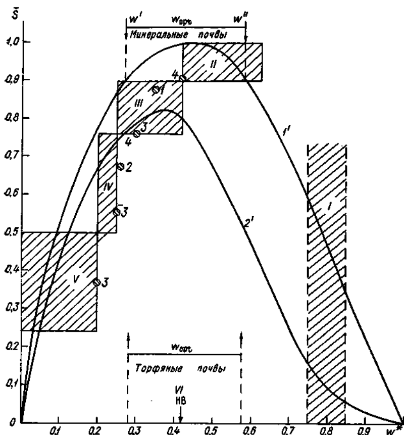
Рис. 15. Сравнение теоретических кривых \bar{S}(w^*) с экспериментальными данными по критическим влажностям и оптимальным для растений диапазонам.
