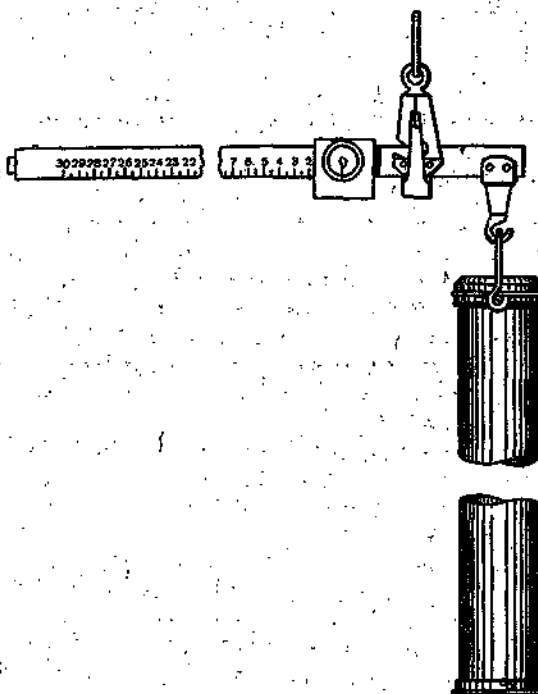
Рис. 27. Снегомер весовой.
