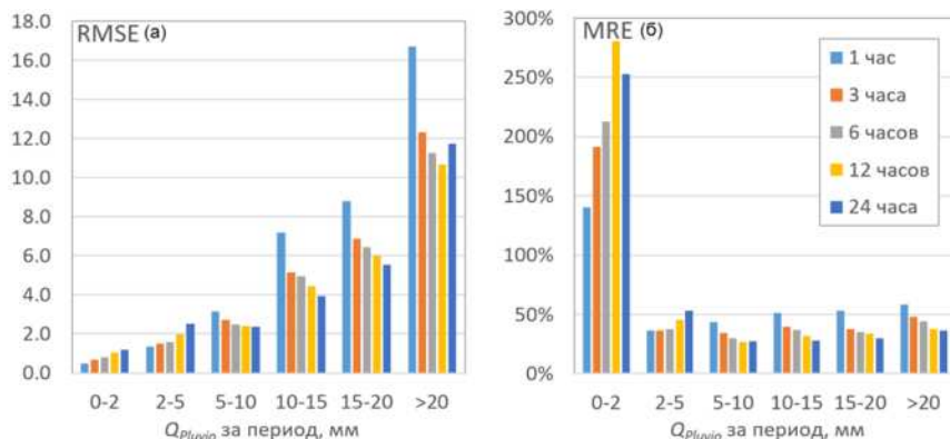
Рисунок 3 – Гистограммы распределения среднеквадратической (а) и относительной (б) ошибок измерения количества осадков
