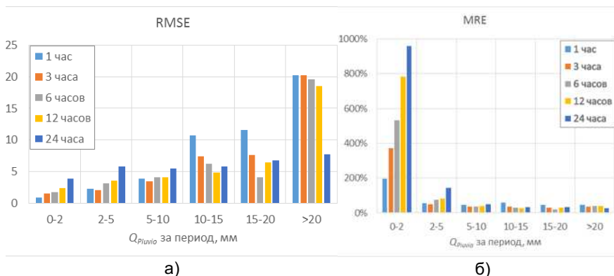
Рисунок 3 – Гистограммы распределения среднеквадратической (а) и относительной (б) ошибок измерения количества осадков
