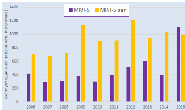
Рисунок 2. Динамика средней годовой эксплуатационной надежности МРЛ за 2006 – 2015 гг.
