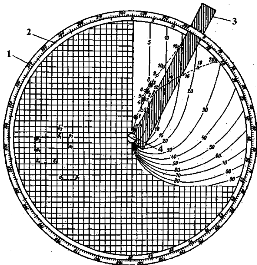
Рис. 3.1. Планшет Молчанова для графической обработки данных одноpunktных шар-пилотных наблюдений (планшет аэрологический А-30):
