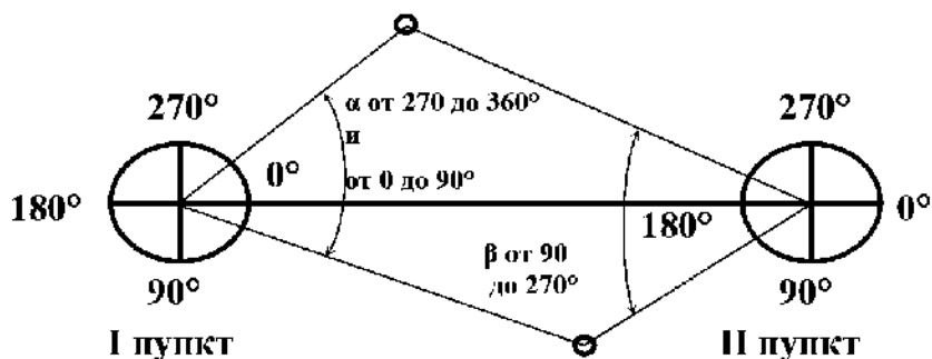
Рис. 5.11. Значения горизонтальных углов при положении проекции шара между пунктами базы
