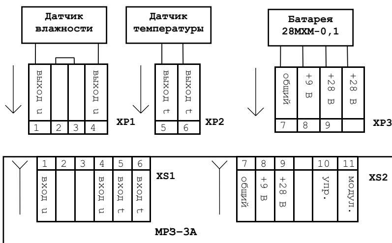
Рис. 6.7. Соединение датчиков температуры, влажности и источника питания с радиозондом МРЗ-3а
