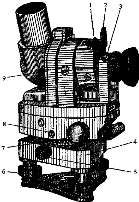
Рис. 2.5. Теодолит 2АШТ со стороны окуляра: 1, 2 – рукоятки; 3 – лампа; 4 – подставка; 5 – зажимной винт; 6 – подъёмный винт; 7 – горизонтальный наводящий винт; 8, 9 – резьбовые пробки
