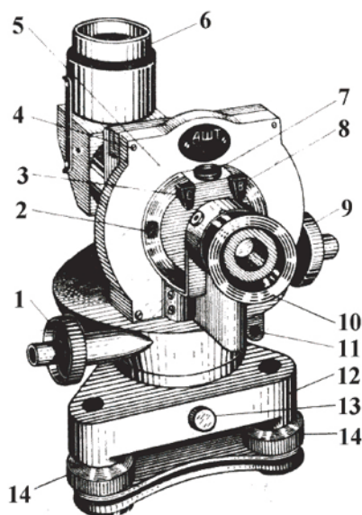
Рис. 2.2. Общий вид теодолита АШТ:
