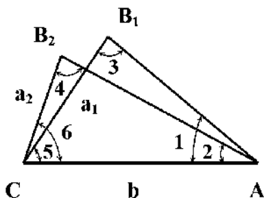
Рис. 5.3. Измерение базы с помощью треугольников, расположенных по одну сторону базисной линии
