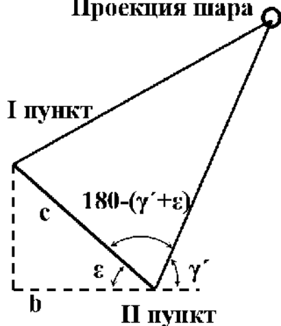
Рис. 5.14. Значение угла (\gamma' \pm \varepsilon) при первом положении пунктов. Случай 3. Горизонтальные углы \alpha < 90^\circ или \alpha > 270^\circ и \beta < 90^\circ или \beta > 270^\circ |\gamma' + \varepsilon|
