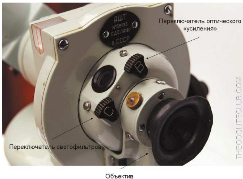
Рис. 2.1 (Окончание). Внешний вид и детали аэрологического теодолита
