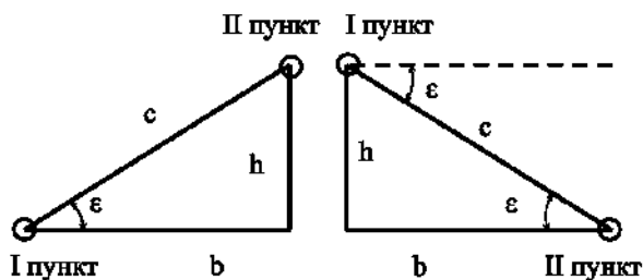
Рис. 5.4. Две схемы взаимного расположения двух пунктов наблюдения и соответствующее определение: длины базы b , расстояния между пунктами базы c , превышение одного пункта над другим h и угол превышения \varepsilon
