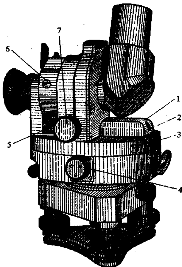
Рис. 2.6. Теодолит 2АШТ со стороны объектива: 1, 5 – крышки; 2 – винт; 3, 6 – пробки; 4 – рукоятка перевода лимба горизонтального круга; 7 – вертикальный наводящий винт
