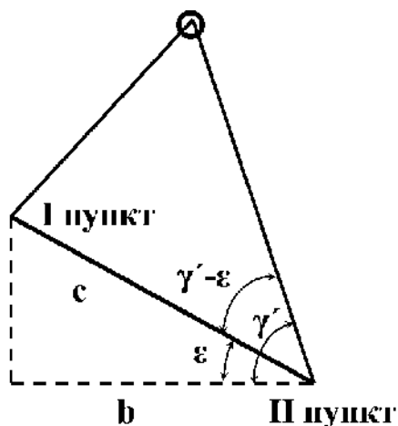
Рис. 5.12. Значение угла (\gamma' \pm \varepsilon) при первом положении пунктов. Случай 1. Горизонтальные углы \alpha < 90^\circ или \alpha > 270^\circ и 90^\circ < \beta < 270^\circ |\gamma' - \varepsilon|
