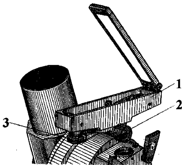
Рис. 2.9. Ориентир-буссоль:
