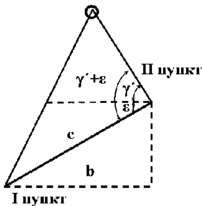
Рис. 5.15. Значение угла (\gamma' \pm \varepsilon) при втором положении пунктов. Случай 1. Горизонтальные углы \alpha < 90^\circ или \alpha > 270^\circ и 90^\circ < \beta < 270^\circ |\gamma' + \varepsilon|
