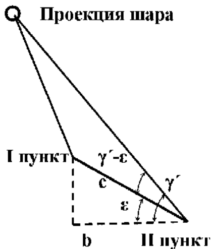
Рис. 5.13. Значение угла (\gamma' \pm \varepsilon) при первом положении пунктов. Случай 2. Горизонтальные углы 90^\circ < \alpha < 270^\circ и 90^\circ < \beta < 270^\circ |\gamma' - \varepsilon|
