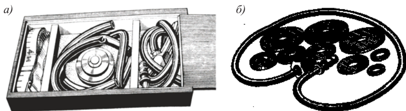
Рис. 1.2. Шар-пилотный комплект ШК-50: а) общий вид; б) резиновый шланг с разновесами
