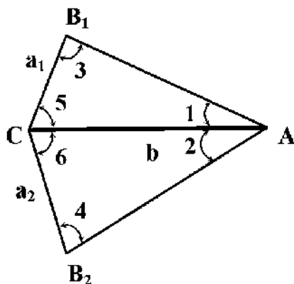
Рис. 5.2. Измерение базы с помощью косоугольных треугольников
