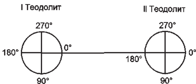
Рис. 5.5. Схема установки теодолитов на концах базы
