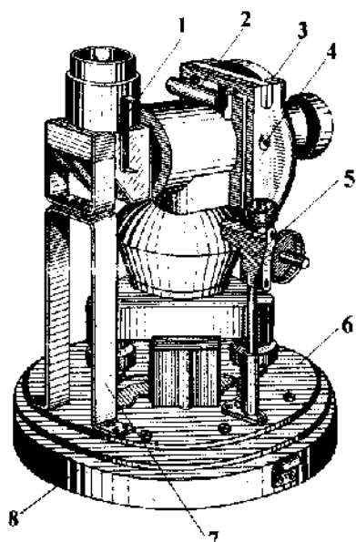
Рис. 2.3. Теодолит АШТ с установочным основанием:
