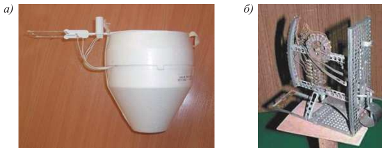
Рис. 6.1 Радиозонды: а – внешний вид радиозонда МРЗ-Зак; б – механическая часть радиозонда Молчанова
