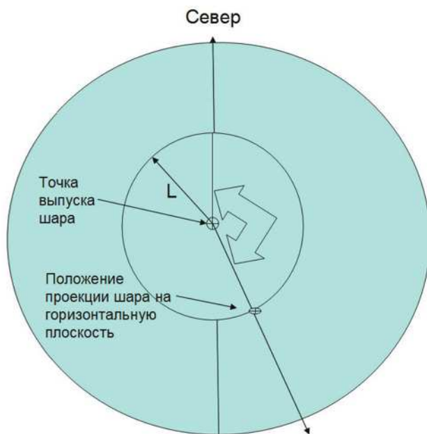
Рис. 3.2. Схема определения положения проекции шар-пилота на горизонтальную плоскость графическим методом: L – удаление проекции шар-пилота от точки выпуска (от центра круга), двойной стрелкой указано значение горизонтального угла
