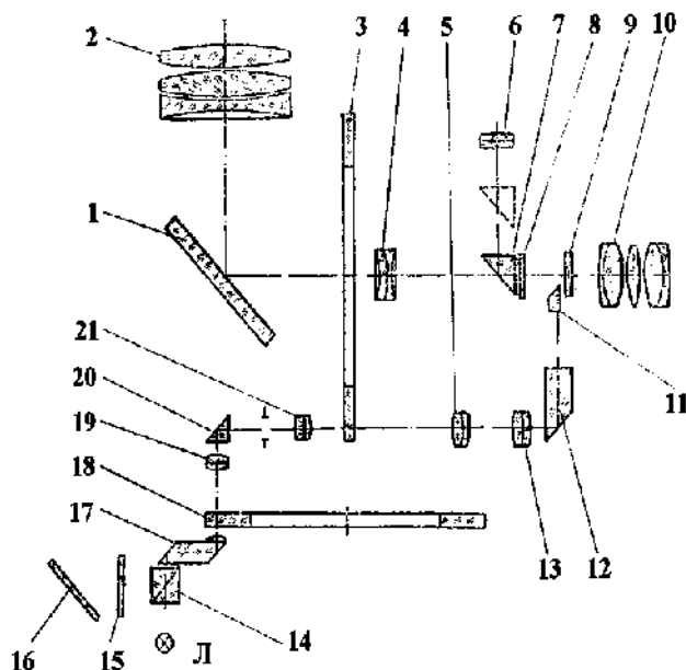
Рис. 2.7. Оптическая схема теодолита 2АШТ: 1 – зеркало; 2 – объектив; 3 – вертикальный круг; 4 – фокусирующая линза; 5, 13, 19, 21 – линзы; 6 – объектив визира; 7 – подвижная призма; 8 – сменный светофильтр; 9 – сетка; 10 – окуляр; 11, 12, 20 – призмы; 14 – призма-куб; 15 – иллюминатор; 16 – поворотное зеркало; 17 – призма с коллективом; 18 – горизонтальный круг, Л – лампа
