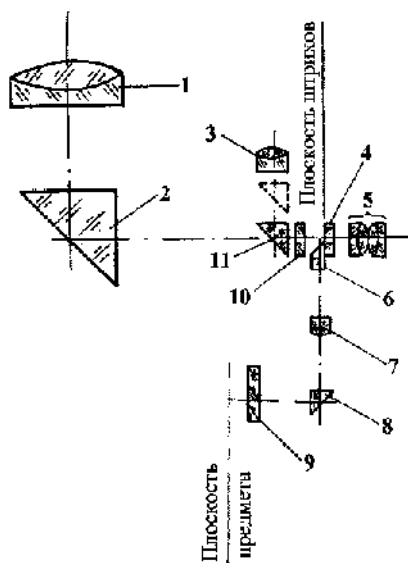
Рис. 2.4. Оптическая схема теодолита АШТ: 1 – объектив зрительной трубы; 2, 6, 8, 11 – призмы; 3 – объектив визира; 4 – сетка; 5 – окуляр; 7 – объектив отсчётной системы; 9 – защитное стекло; 10 – светофильтр
