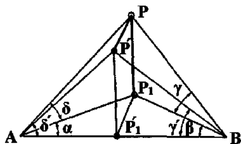
Рис. 5.7. Проекция шара-пилота и визирных линий на горизонтальную и вертикальную плоскости
