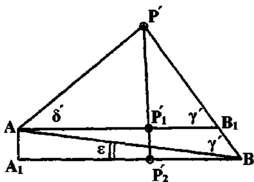
Рис. 5.8. Проекция шара-пилота и визирных линий на вертикальную плоскость при разных высотах пунктов базы
