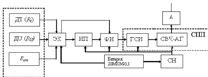
Рис. 6.2. Функциональная схема радиозонда МРЗ-3а (обозначения в тексте)
