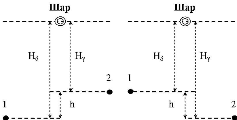
Рис. 5.10. Высота шара H_\delta и H_\gamma над теодолитами первого и второго пунктов: 1 – уровень первого теодолита; 2 – уровень второго теодолита
