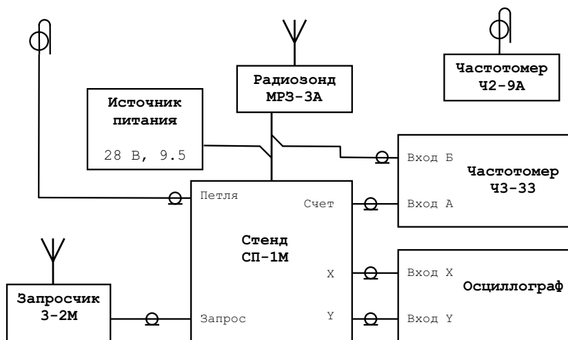
Рис. 6.8 Схема подключения радиозонда МРЗ-3а к КИПАСу
