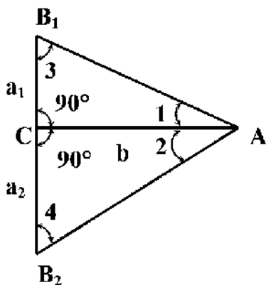
Рис. 5.1. Измерение базы с помощью прямоугольных треугольников
