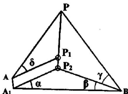
Рис. 5.6. Проекция шара-пилота и визирных линий на горизонтальную плоскость
