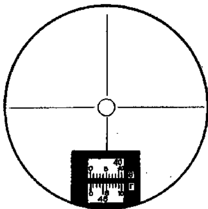
Рис. 2.8. Вид поля зрения отсчётного микроскопа теодолита 2АШТ: отсчёт по вертикальному кругу 40,90^\circ , отсчёт по горизонтальному кругу 46,40^\circ
