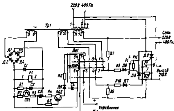
Рис 144 Принципиальная схема РН 0,5
