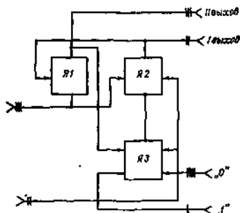
Рис 9.12 Динамический триггер
