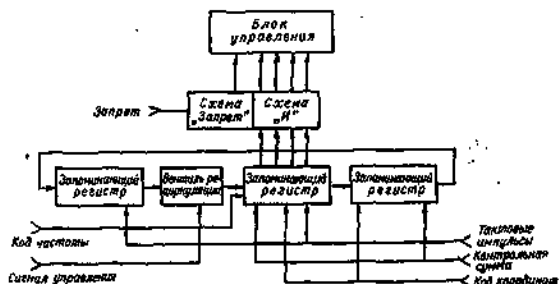
Рис. 9.17. Запоминающий регистр.
