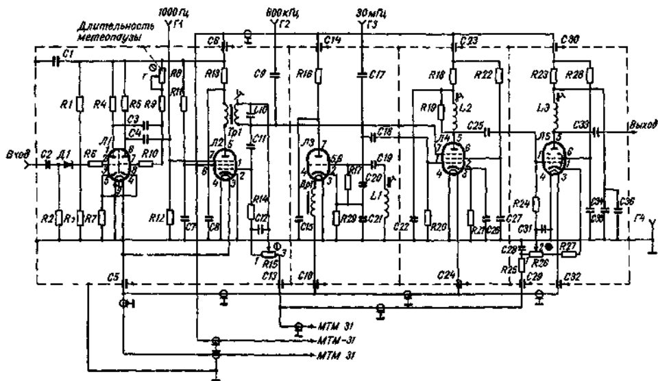
Рис 37 Принципиальная схема устройства встроенного контроля
