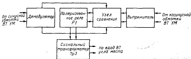
Рис. 19.3. Блок-схема линейки сканирования.
