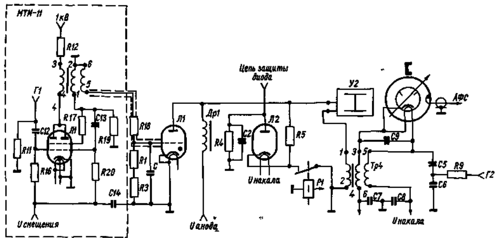
Рис 24 Принципиальная схема передатчика большой мощности
