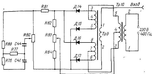
Рис 5.14 Демодулятор обратной связи
