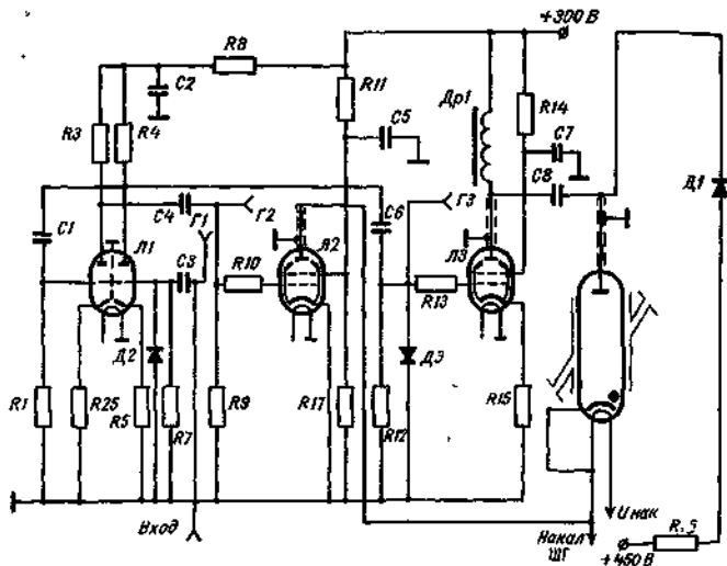
Рис 165. Модулятор генератора шума.
