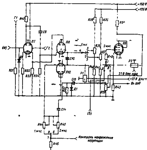
Рис 15.12 Принципиальная схема тинення сложения (продолжение)
