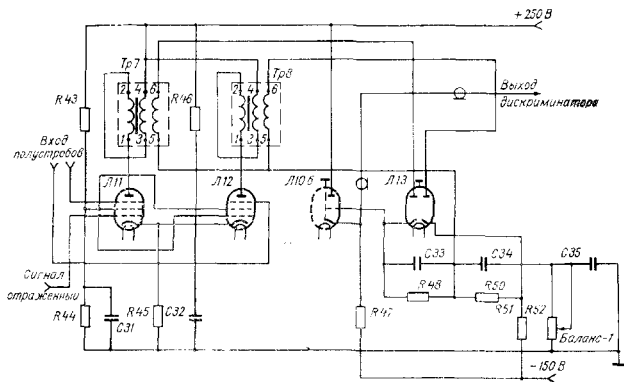
Рис. 5.12. Схема формирования сигнала ошибки.
