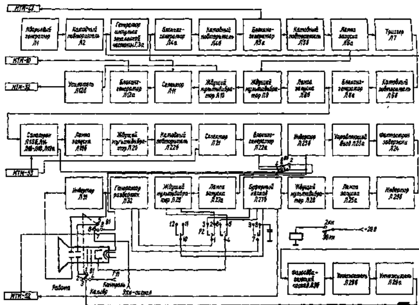
Рис 51. Функциональная схема блока МТМ-51.
