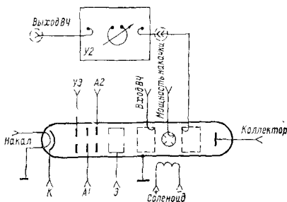
Рис. 34 Принципиальная схема электронного параметрического усилителя.
