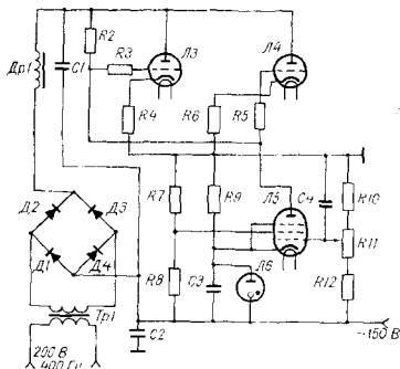
Рис. 8.2. Стабилизированный выпрямитель -150 В, 140 мА.
