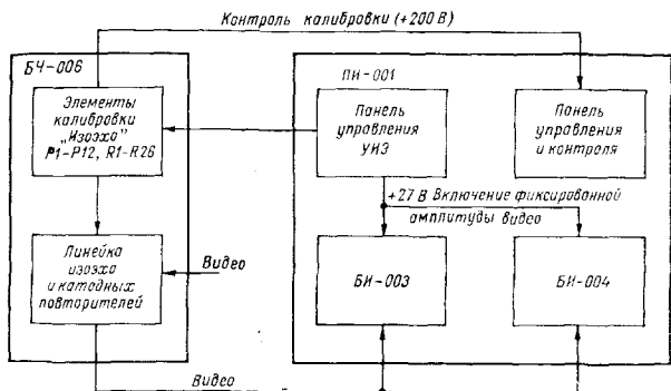
Рис. 18.2. Функциональная схема устройства «Изоэхо».
