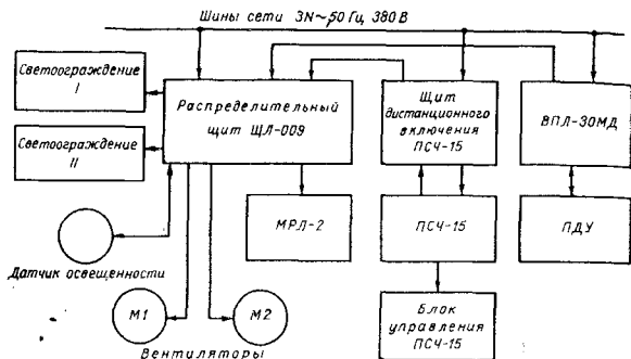
Рис. 20.1. Блок-схема электроснабжения.
