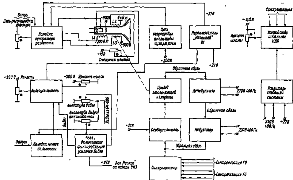
Рис. 175 Функциональная схема ИДВ.
