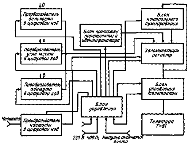
Рис 91 Блок-схема устройства «ОКА-3»
