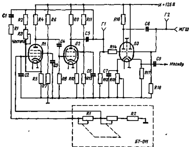
Рис. 16.2. Задающий генератор.
