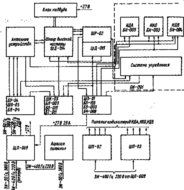
Рис. 12.1. Функциональная схема МРЛ-2.
