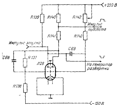
Рис. 5.7. Генератор 30-км строба
