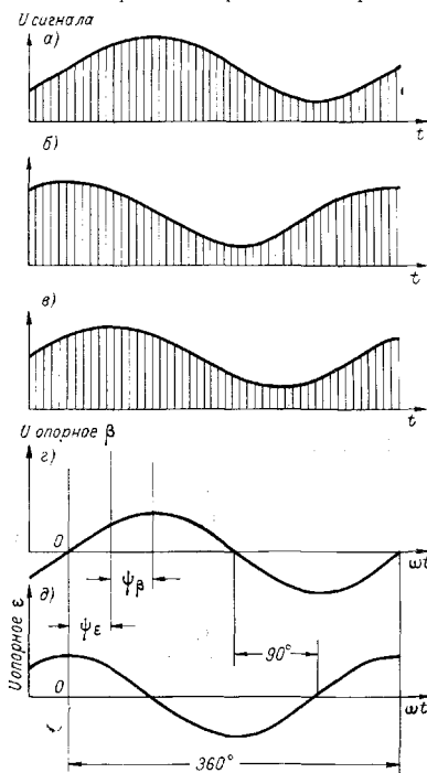
Рис. 7.3. Фазы сигнала ошибки при различных отклонениях электрической оси антенны от направления на цель.
