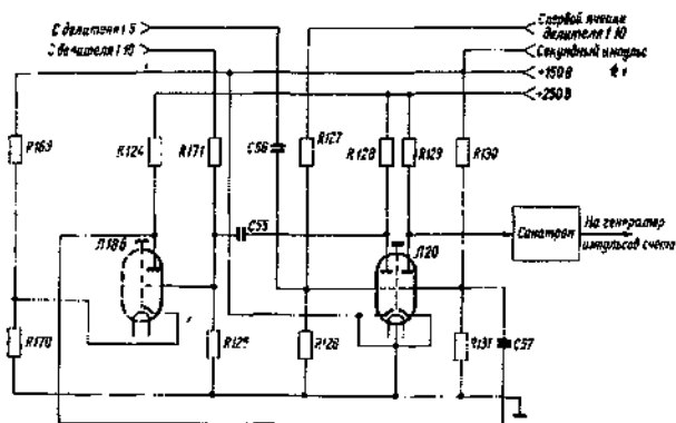
Рис 4.9 Схема формирования задержки
