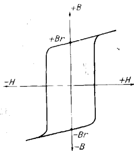
Рис. 9.2б. Прямоугольная петля гистерезиса.
