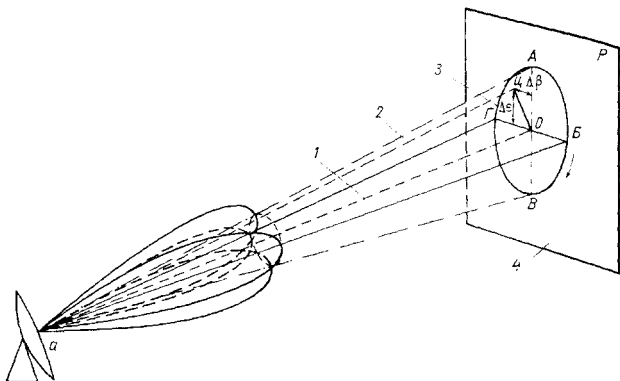
Рис. 7.1. Коническое разворачивание луча диаграммы направленности.
