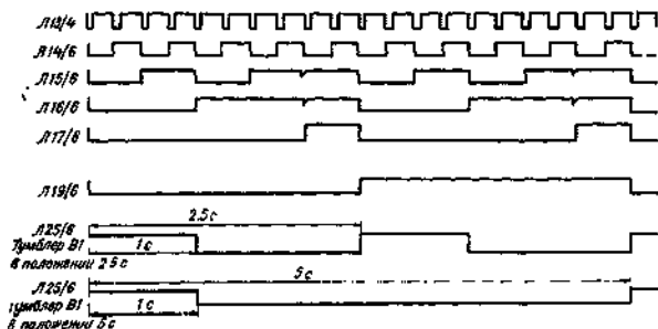
Рис 4.8 Эпюры напряжений.
