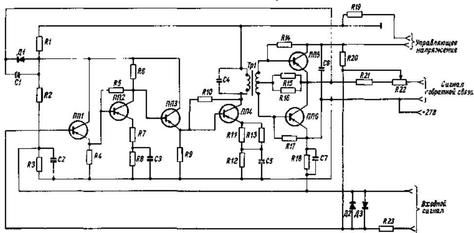
Рис 17 14 Принципиальная схема усилителя следящей системы
