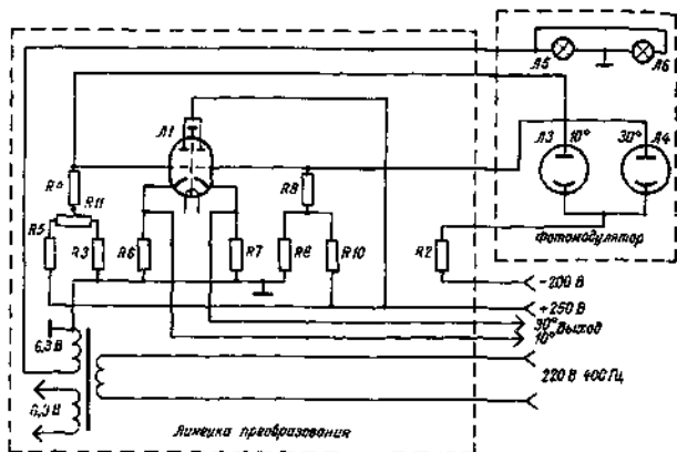
Рис. 19.2. Схема преобразования импульсов фотомодулятора.
