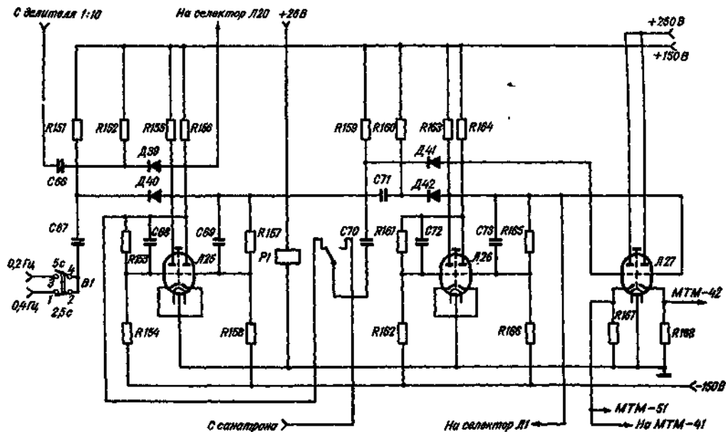
Рис 47. Принципиальная схема формирования импульса счета.
