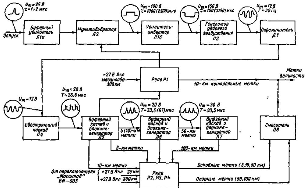
Рис. 17.4. Функциональная схема линейки меток дальности.
