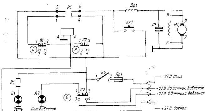
Рис. 13.4. Принципиальная схема блока наддува.
