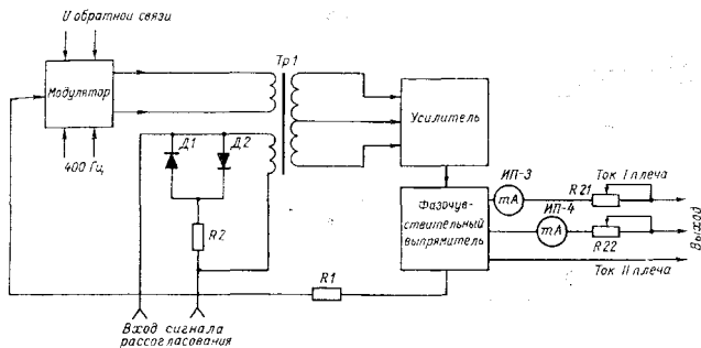
Рис. 19.5. Функциональная схема полупроводникового усилителя.
