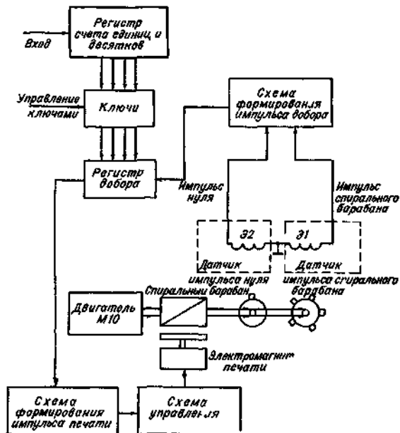
Рис 63 Схема регистрации метеоуказаний разряда единиц и десятков
