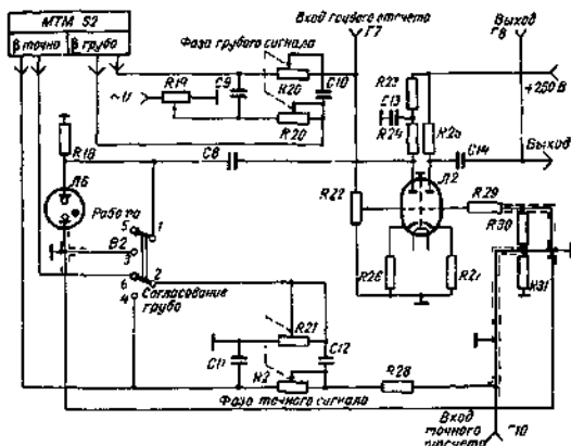
Рис 64 Принципиальная схема СУД канала азимута
