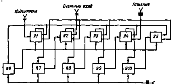
Рис 9 13 Счетчик
