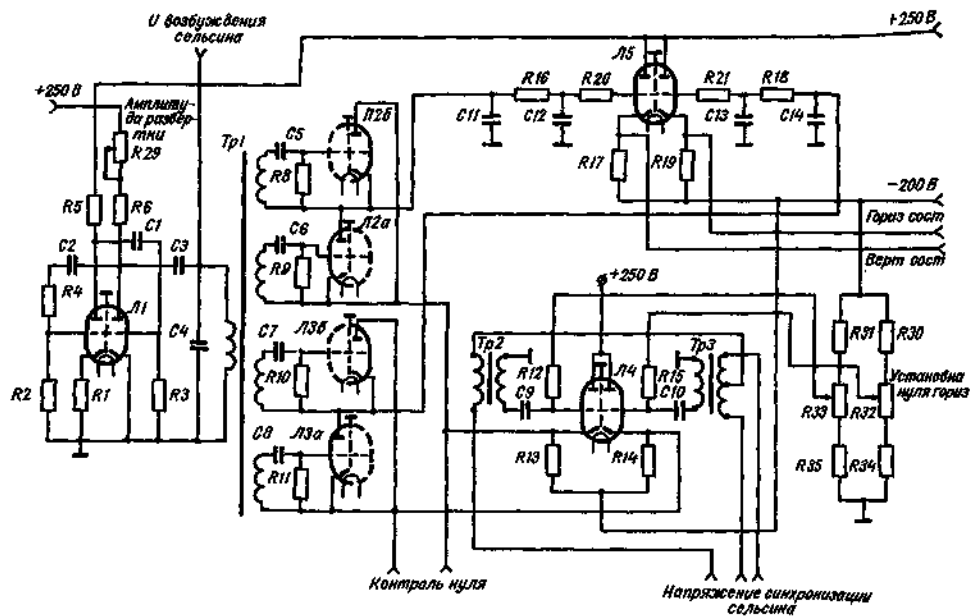
Рис 185 Принципиальная схема линенки датчика развсртыивающих напряжений
