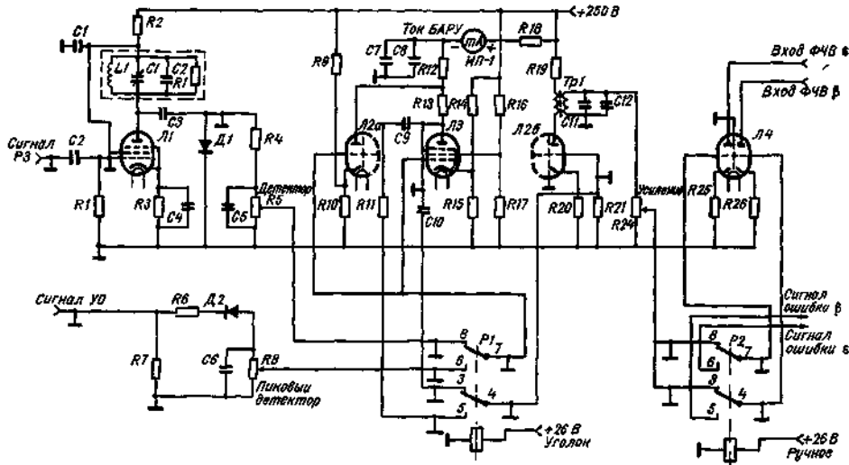
Рис 78 Принципиальная схема формирования сигнала ошибки.
