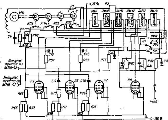
Рис. 6.8. Схема управления печатающим устройством.
