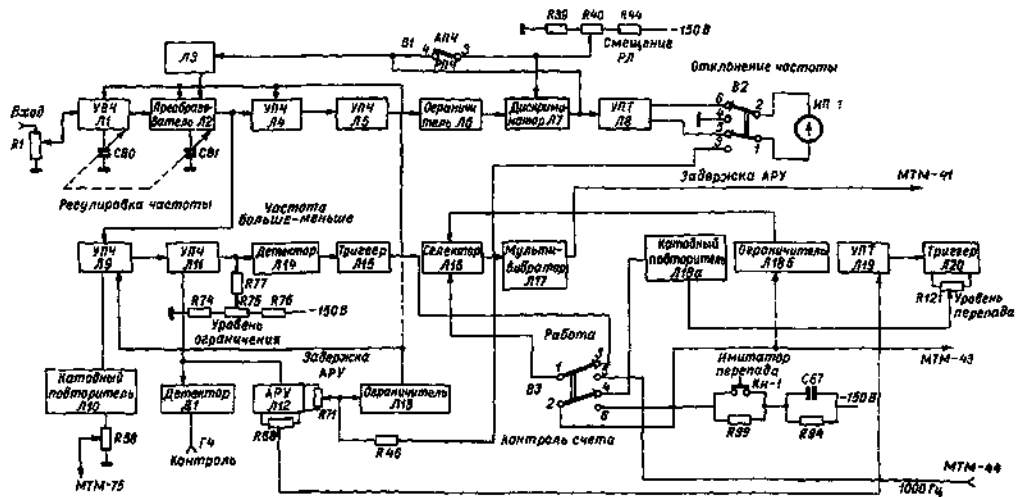
Рис 33 Функциональная схема блока МТМ 33
