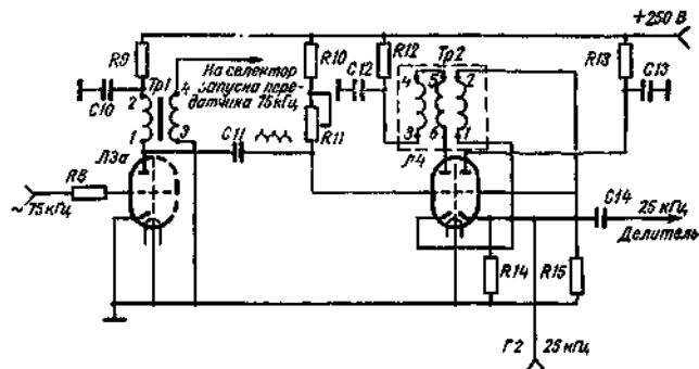
Рис. 5.5 Принципиальная схема генератора импульсов эталонной частоты и первого делителя
