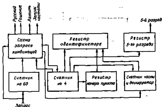
Рис. 9.19. Функциональная схема блока автоматической протяжки перфоленки и перфорации идентификатора части.
