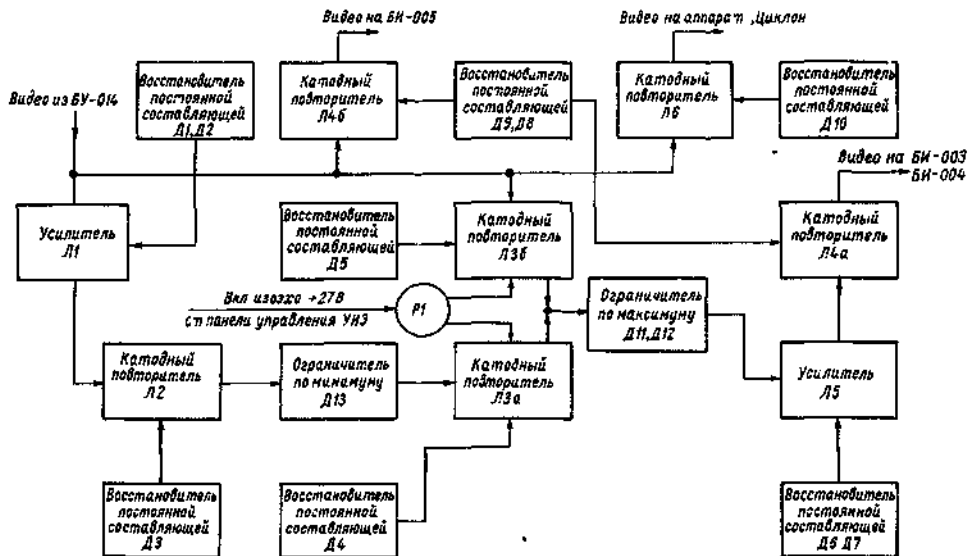
Рис 183 Функциональная схема линейки изозко и катодных повторителей
