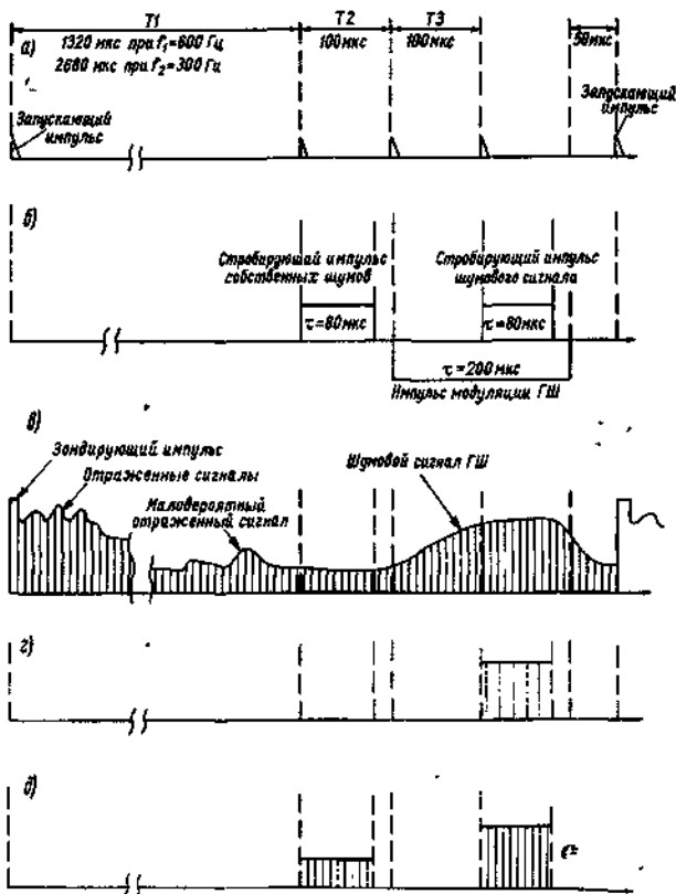
Рис. 15.2. Временные диаграммы работы АСУ, контроля усиления и чувствительности.
