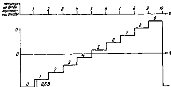
Рис. 4.13. Эпюры напряжений на выходе измерительной схемы
