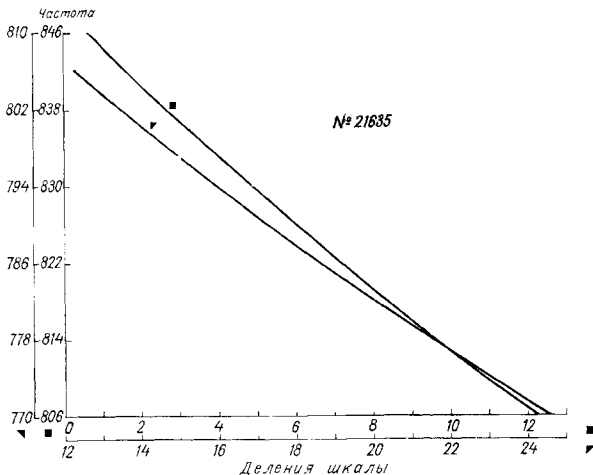
Рис. 10.2. График перевода частоты в деления шкалы контрольного резонатора.
