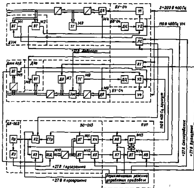
Рис. 19.1. Функциональная схема электропривода.
