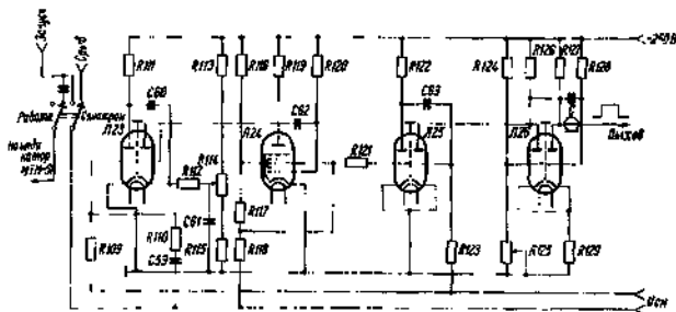
Рис. 5.8. Генератор 2-км строба.
