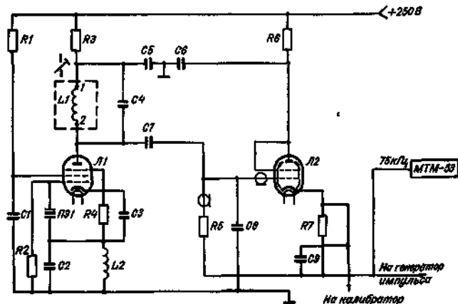
Рис. 54. Принципиальная схема кварцевого генератора.
