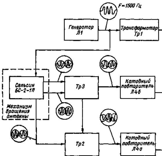
Рис 184 Функциональная схема линенки датчика развертывающих
