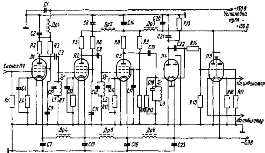
Рис 15.7 Принципиальная схема линейки контроля ПЧ
