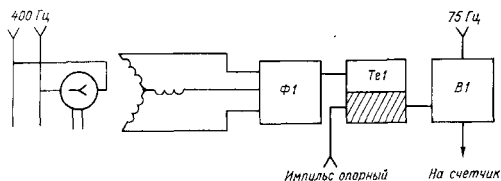
Рис. 9.16. Канал преобразователя.
