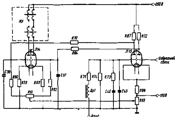
Рис. 5.13. Усилитель постоянного тока.
