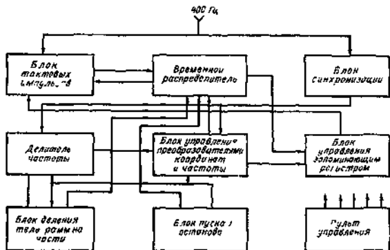
Рис 9.20 Блок-схема устройства управления
