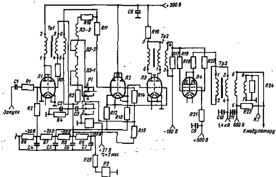
Рис. 14.2. Принципиальная схема подмодулятора.
