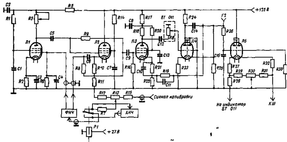
Рис. 16.4 Усилитель низкой частоты
