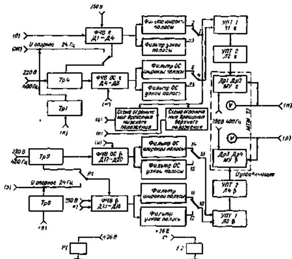
Рис 75 Функциональная схема блоков МТМ 72 и МТМ 73
