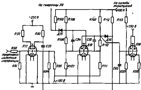
Рис. 4.15 Принципиальная схема формирования импульсов изменения информации.
