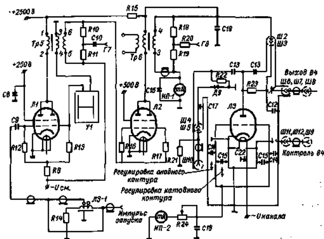
Рис. 2.3. Принципиальная схема передатчика малой мощности.
