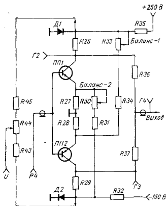
Рис. 5.16. УПТ-1.
