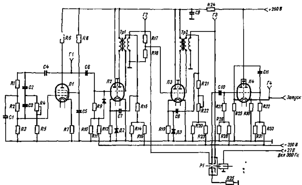
Рис 18 | Принципиальная схема линейки запуска
