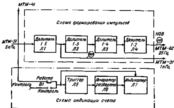
Рис. 4.4. Функциональная схема блока МТМ-44.
