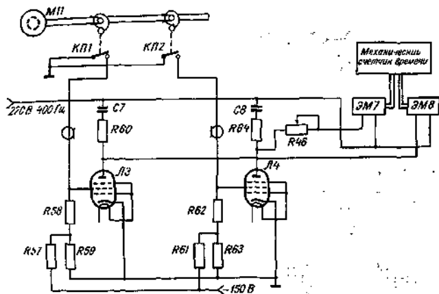
Рис 6.7. Схема набора времени.
