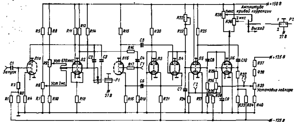
Рис. 15.10. Принципиальная схема линейки коррекции.
