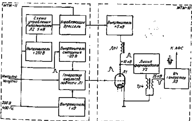
Рис. 2.2. Функциональная схема передатчика большой мощности.
