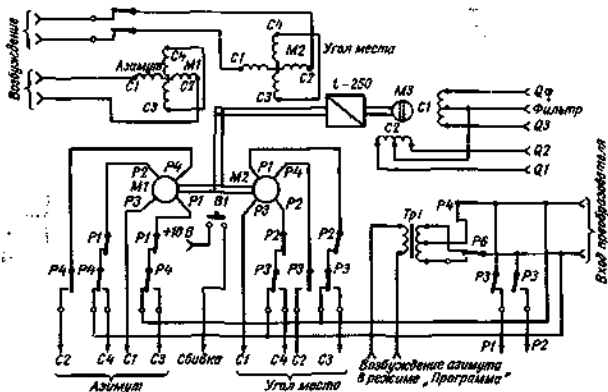
Рис. 19.6. Упрощенная принципиальная схема блока программного устройства.
