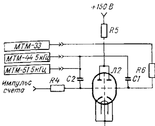
Рис. 4.5. Принципиальная схема селектора 1 блока МТМ-43.
