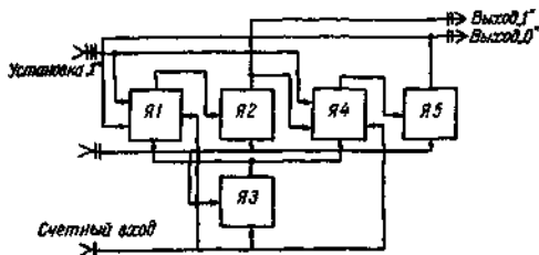
Рис 9.11 Триггер
