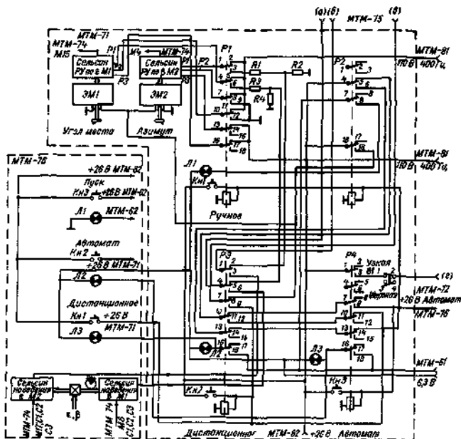
Рис. 7.4. Функциональная схема блоков МТМ-71 и МТМ-76.
