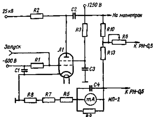
Рис. 14.3 Принципиальная схема модулятора.
