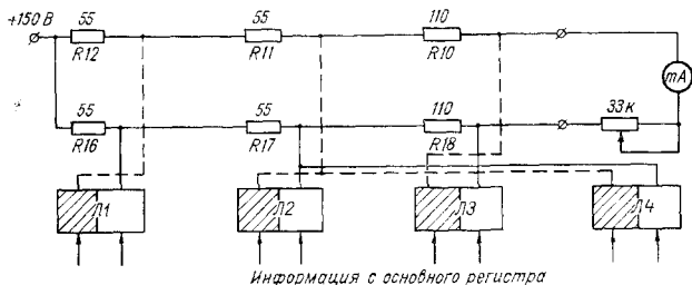
Рис. 4.12. Измерительная схема декады единиц контрольного регистра.
