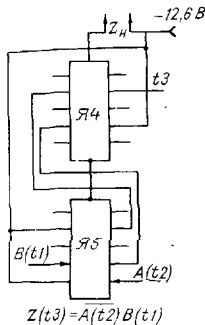
Рис. 9.6. Логический элемент «Запрет».
