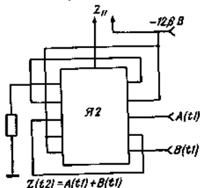
Рис. 9.4. Логический элемент «Или» с подмагничиванием.
