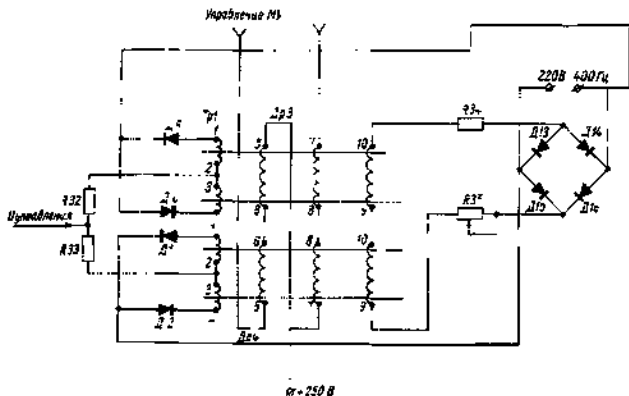
Рис 6.6 Магнитный усилитель
