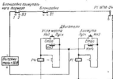
Рис. 8.4. Схема блокировки приводных двигателей антенной колонки.
