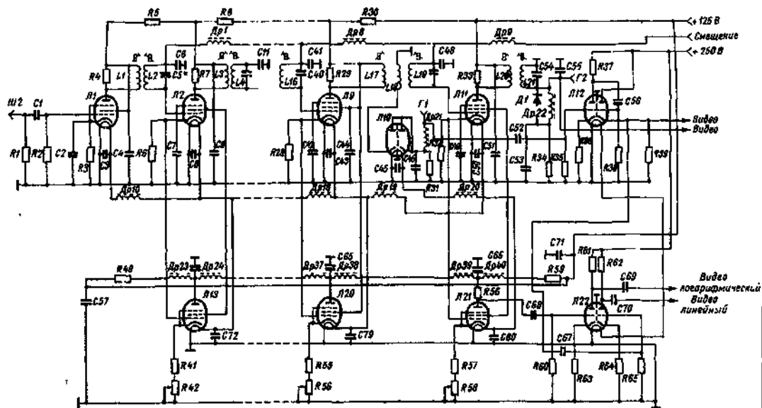
Рис 159 Принциальная схема УПЧ с ЛАХ.
