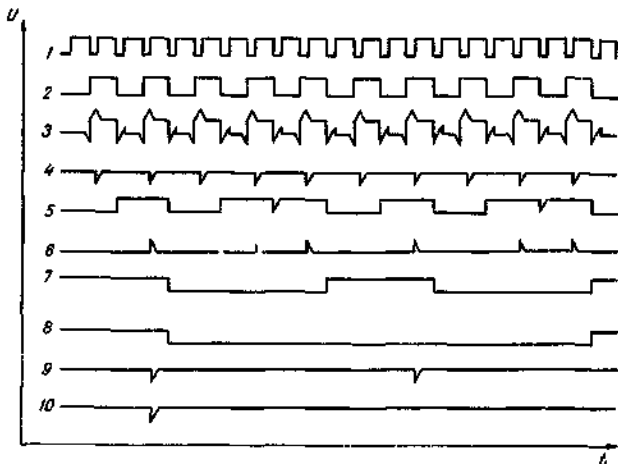
Рис. 4.10. Эпюры напряжений схемы формирования задержки.
