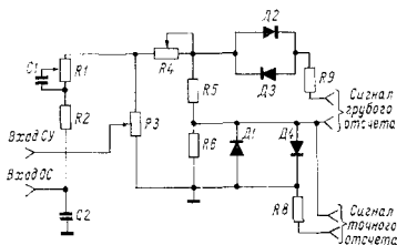
Рис. 17.10. Синхронизатор.
