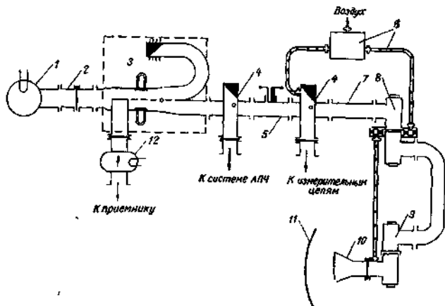
Рис 13.1 Функциональная схема антенно волноводной системы
