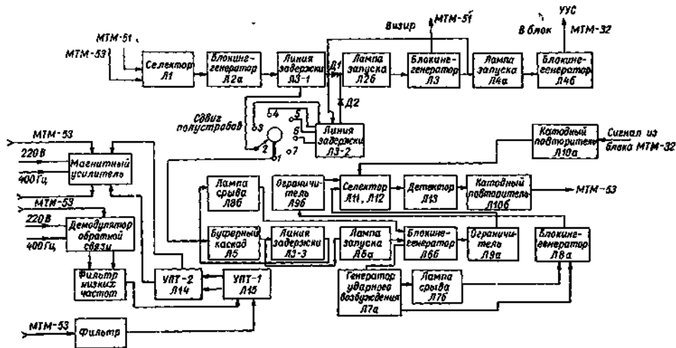
Рис. 5. 2. Функциональная схема блока MTM-52.
