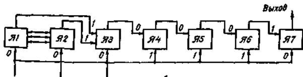
Рис 9 14 Схема синхронизации
