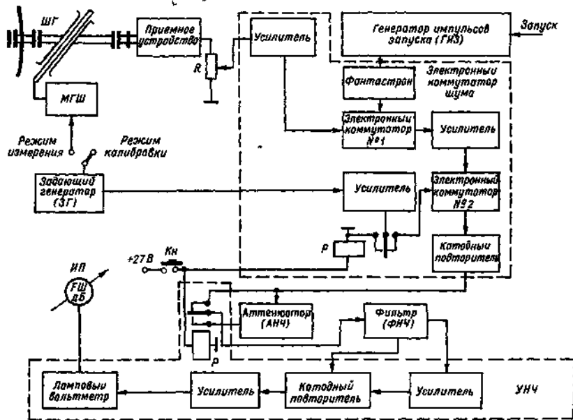
Рис 161 Функциональная схема ЕКС
