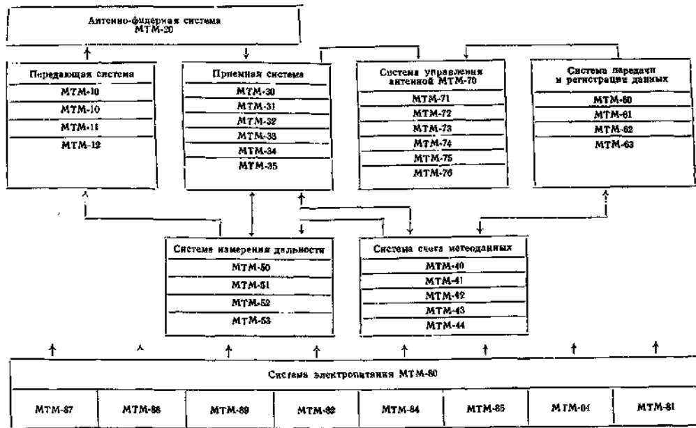
Рис. 1.1. Блок-схема радиолокационной станции «Метеорит-2»
