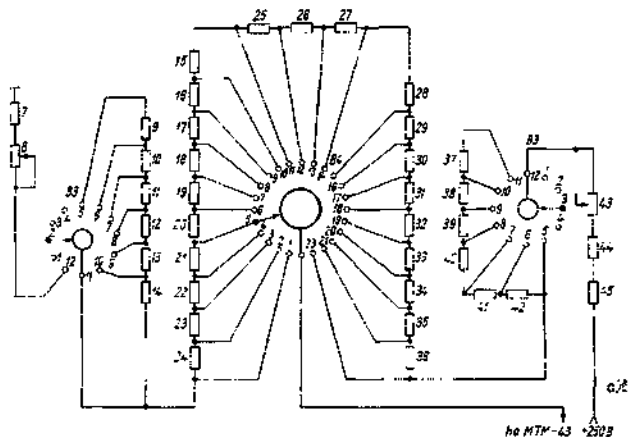
Рис. 6.9. Схема регулировки времени счета.
