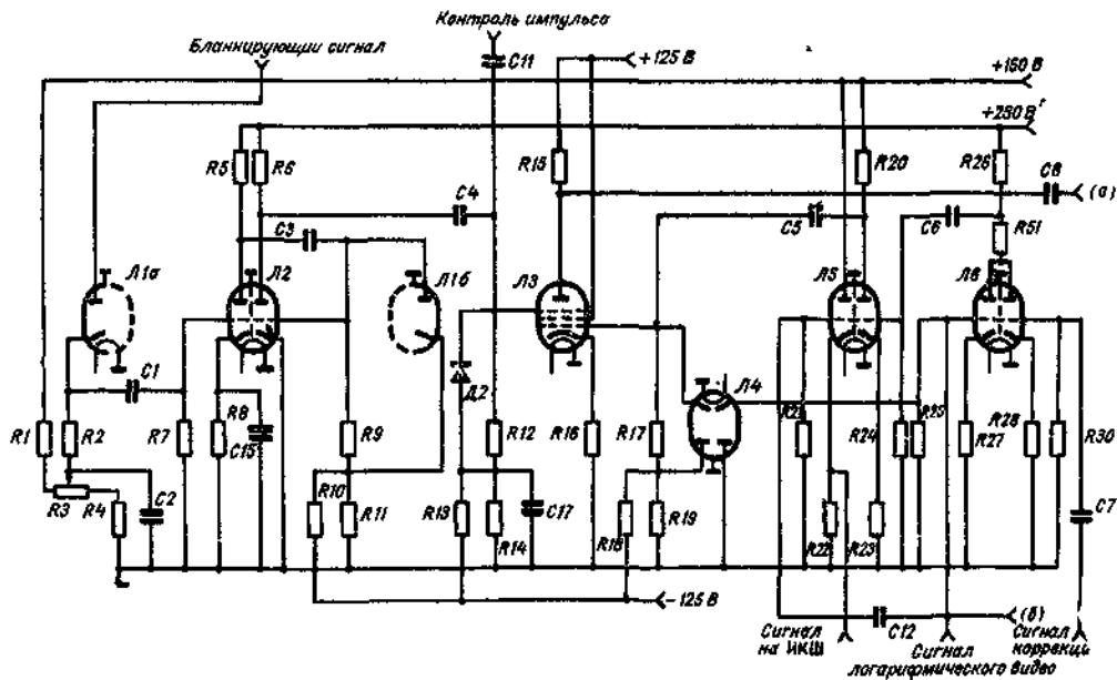
Рис. 15 [1]. Принципиальная схема линейки сложения.
