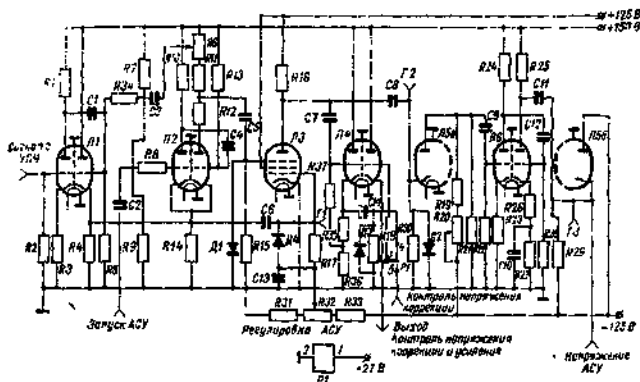
Рис. 15.13. Принципиальная схема линейки АСУ.
