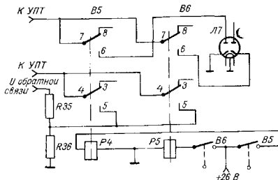
Рис 7 10 Схема ограничения вращения антенной колонки
