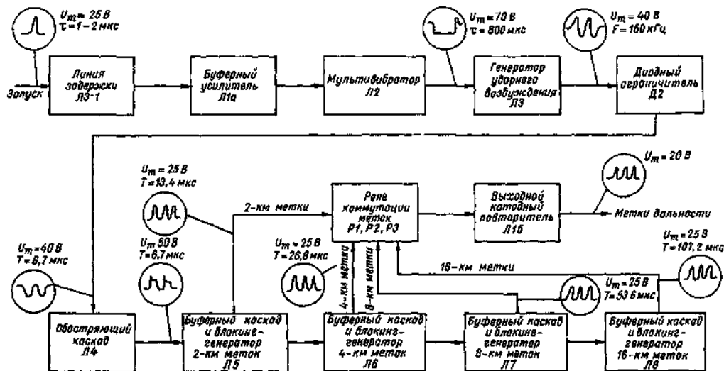
Рис 178 Функциональная схема линейки метода дальности ИДВ
