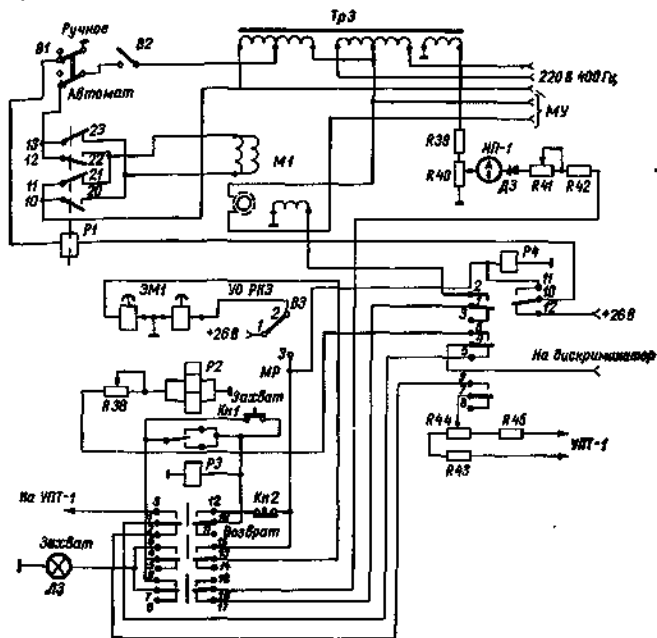
Рис 5.17 Принципиальная схема автозахвата метеоро ракеты
