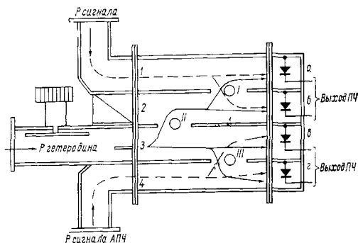
Рис 153 Принципиальная схема смесителя
