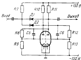
Рис. 4.6. Принципиальная схема пересчетной ячейки делителя.
