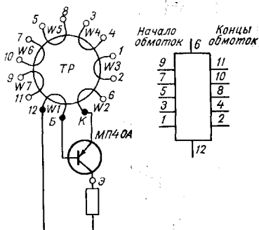
Рис. 9.2а. Ферриттранзисторный модуль.
