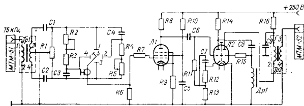
Рис. 5 15. Схема формирования подвижных импульсов.
