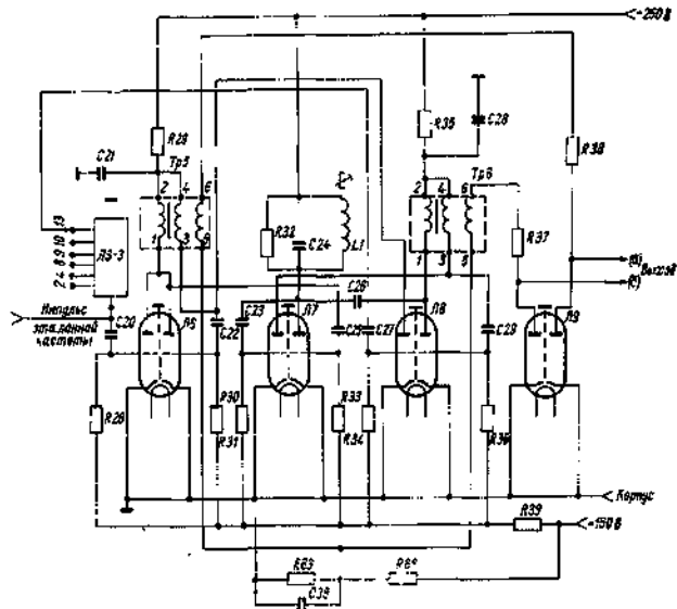
Рис. 5.11. Генератор полустроби.
