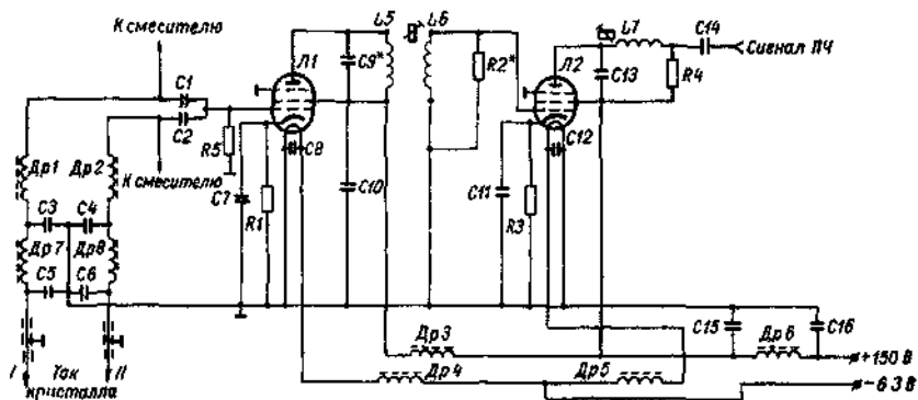
Рис 154 Принципиальная схема ПУПЧ
