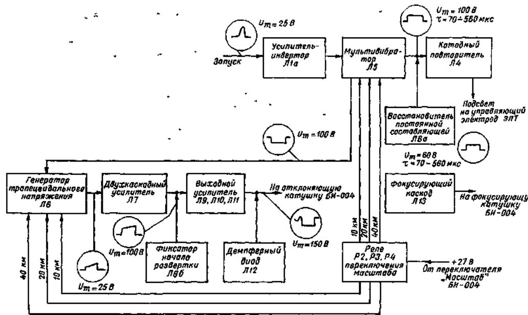
Рис. 176 Функциональная схема линейки генератора развертки ИДВ
