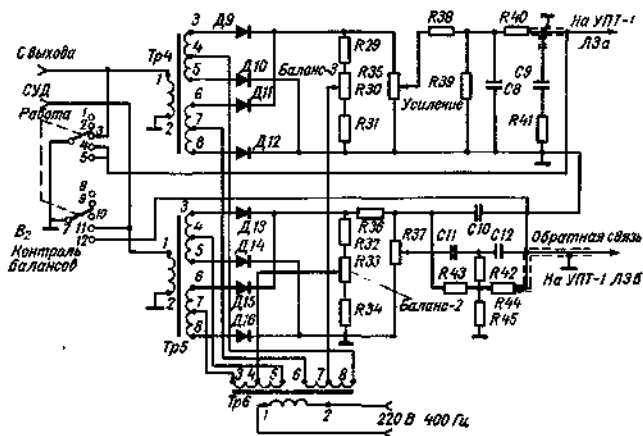
Рис. 6.5 Фазочувствительные выпрямители сигнала ошибки и обратной связи
