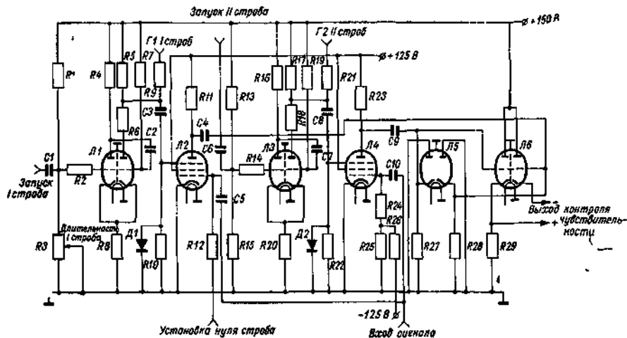
Рис 15.14 Принципиальная схема линейки контроля чувствительности
