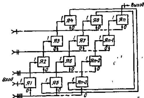
Рис 9.10 Сдвигающий регистр
