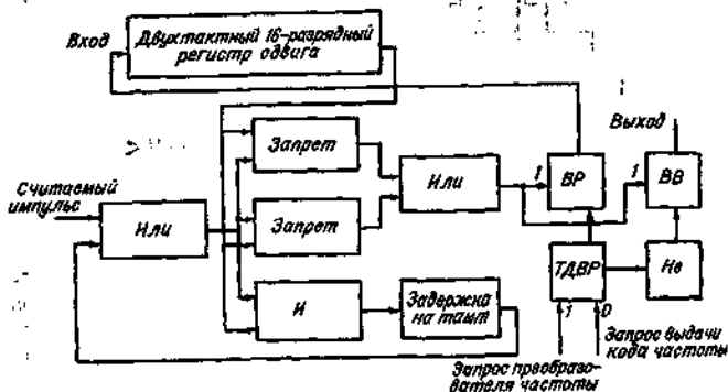
Рис. 9.15. Преобразователь частоты.
