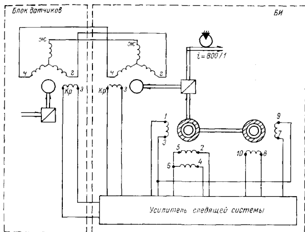
Рис. 17.13. Функциональная схема следящей системы индикации положения.
