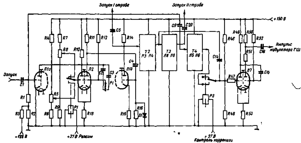
Рис. 15.15 Принципиальная схема линейки временных задержек
