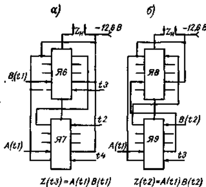
Рис. 9.5. Логический элемент «И»
