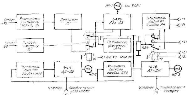
Рис 7.5. Функциональная схема блока МТМ-75.
