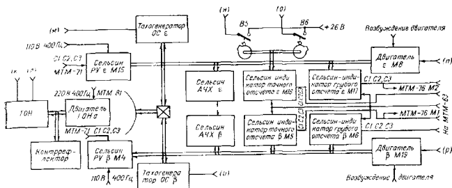
Рис. 7.7. Функциональная схема блока МТМ-74.
