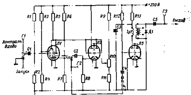
Рис. 16.3. Генератор импульсов запуска
