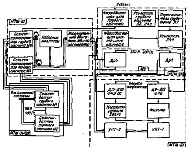
Рис 6.1. Функциональная схема передачи данных.
