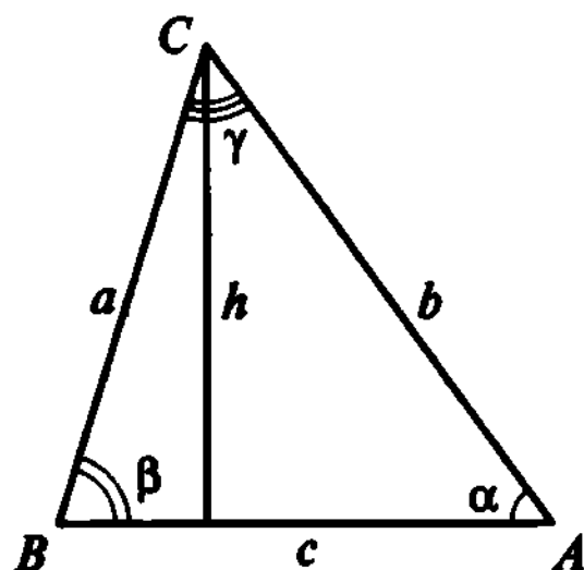
Рис. 2. Треугольник
